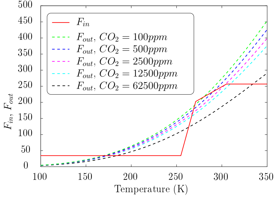
Figure 9: Énergie solaire absorbée par la Terre ( F_{in} ) et énergie infrarouge émise par la Terre ( F_{out} ), en fonction de la température. Les points d'équilibre radiatif correspondent aux points d'intersection entre F_{in}(T) et F_{out}(T) .
