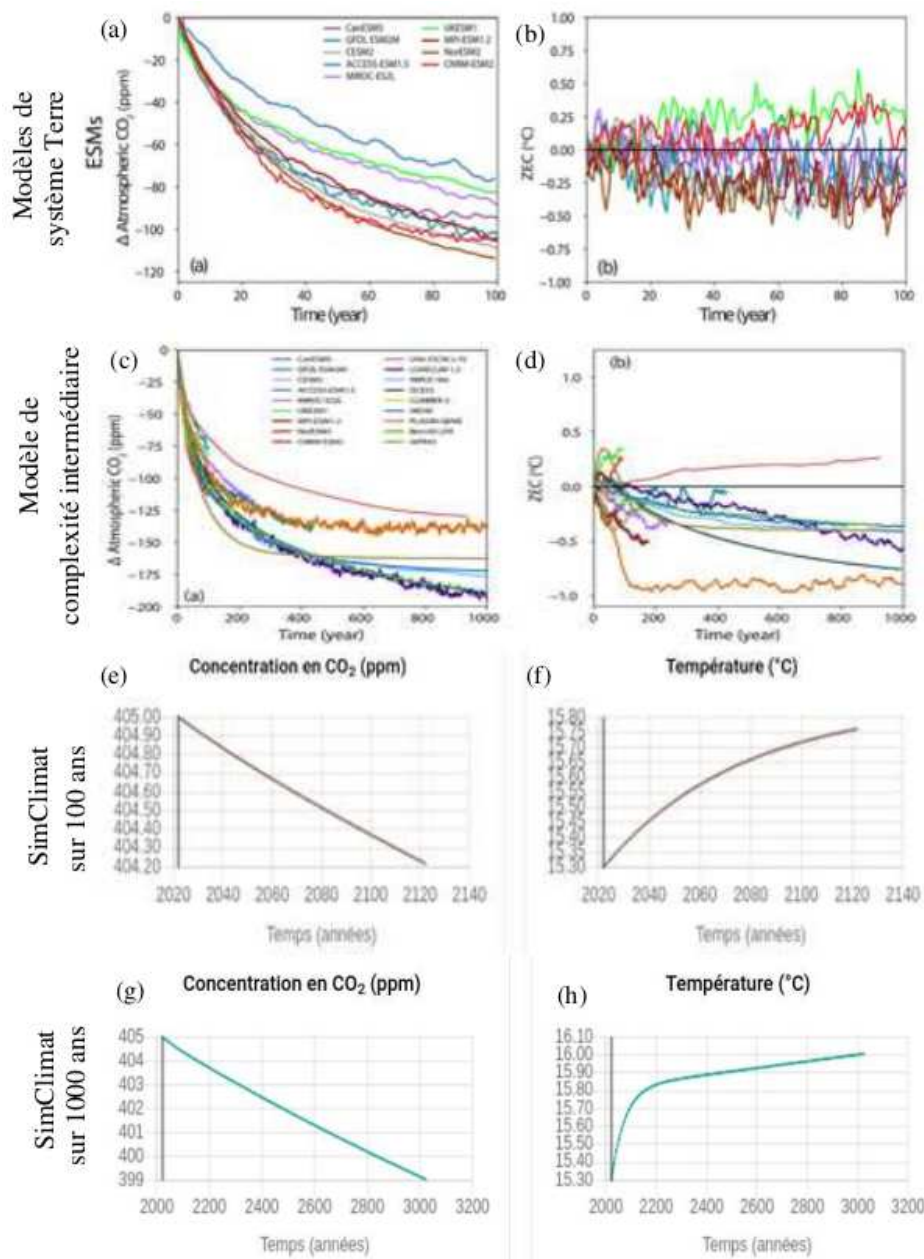
Figure 19: (a) Résultats issus du projet ZECMIP : évolution de la concentration en CO 2 (a, c) et de la température (b, d) au cours du temps après l'arrêt total des émissions, en anomalie par rapport aux valeurs initiales juste avant l'arrêt, simulées sur 100 ans par des modèles de système Terre (a-b) et sur 1000 ans par des modèles de complexité intermédiaire (c-d). Comparaison à ce que donne SimClimat sur 100 ans (e-f) et 1000 ans (g-h) dans les mêmes conditions.
