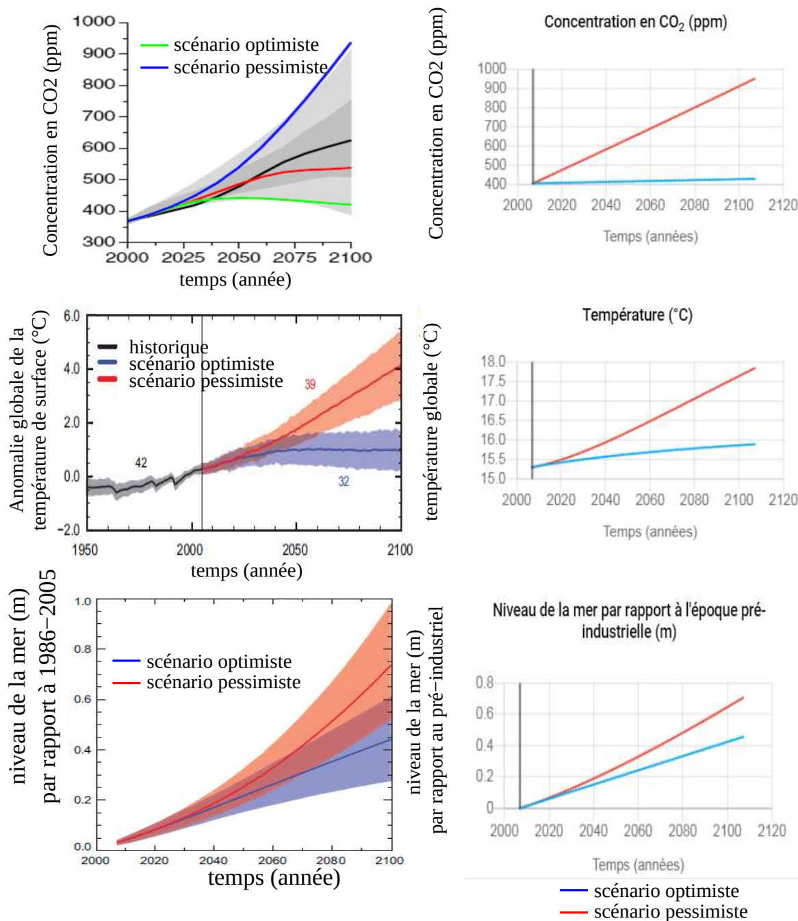
Figure 16: Comparaison des projections produites par SimClimat et par les modèles participant à CMIP. La colonne de gauche présente les résultats montrés dans le 5e rapport du GIEC ([ IPCC, 2013 ]). La colonne de droite montre des captures d'écran de SimClimat. Les courbes montrent l'évolution de la concentration en CO_2 selon des scénarios optimiste et pessimiste (en haut), de la température globale de la Terre (au milieu) et du niveau des mers (en bas). Pour SimClimat, les scénarios optimistes et pessimistes ont été lancés avec des émissions anthropiques de CO_2 de 1 GtC/an et 22 GtC/an respectivement.
