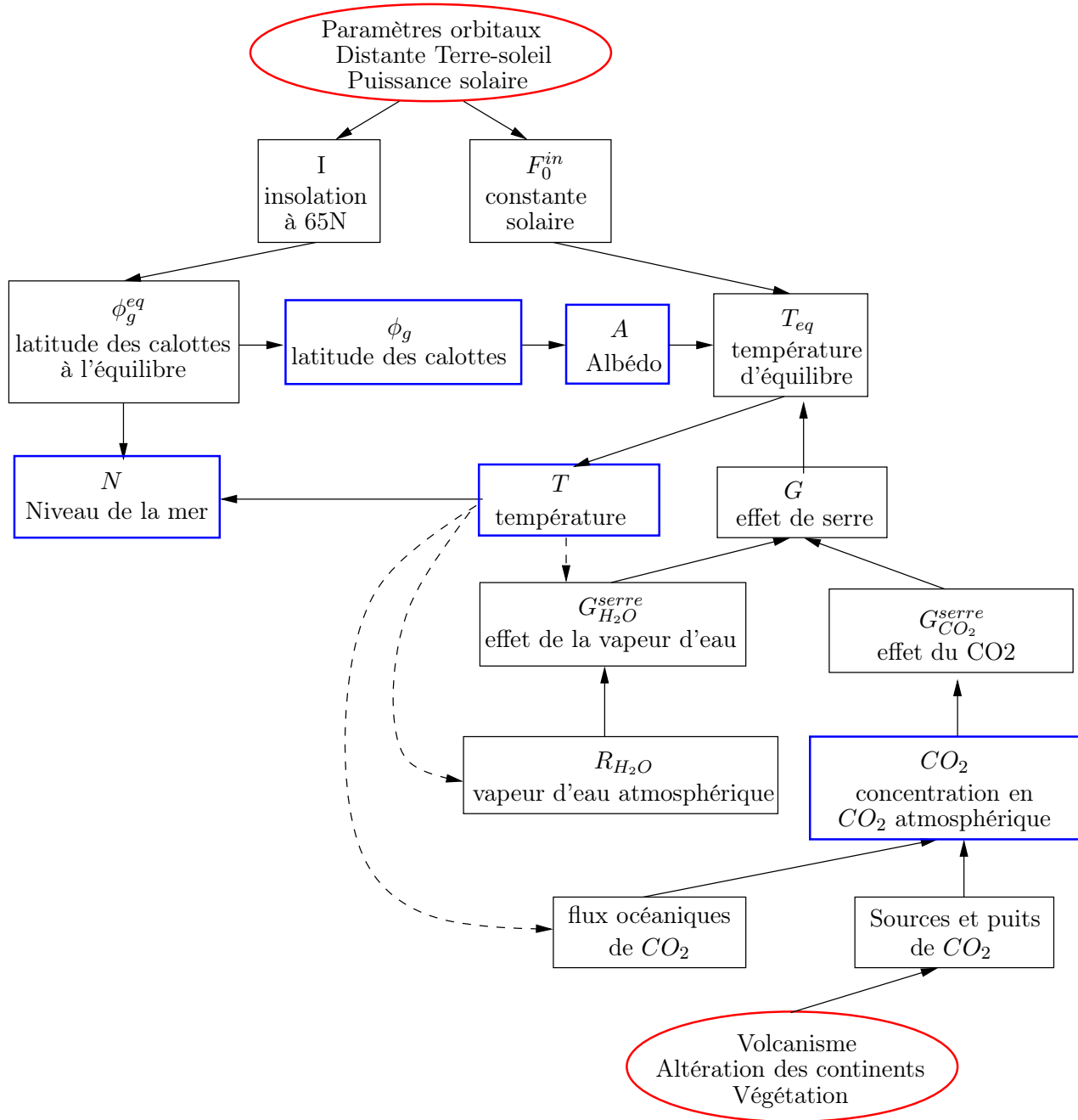
Figure 10: Schéma illustrant comment les différentes variables sont calculées dans le modèle. En rouge: les forçages “externes” au système climatique modélisé. En bleu: les variables d’état du modèle.
