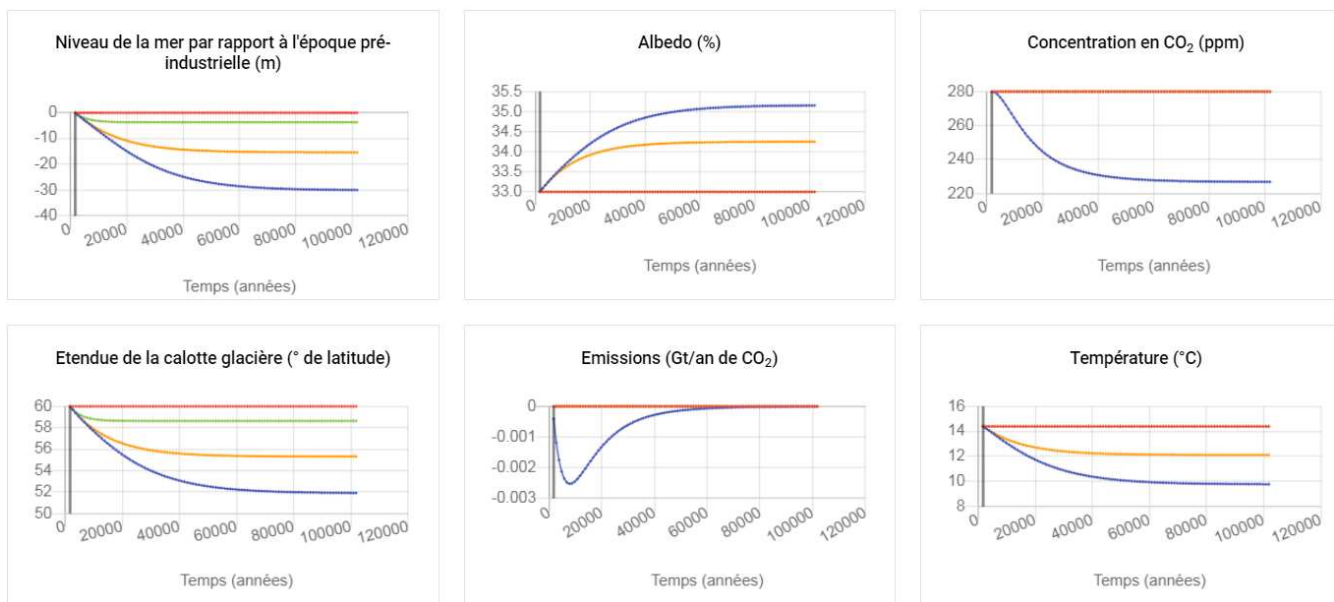
Figure 13: Copie d'écran des résultats d'une simulation pré-industrielle de contrôle de 100 000 ans (rouge), avec une obliquité minimale (bleu), avec obliquité minimale et albédo constant (vert) et avec obliquité minimale et solubilité du CO_2 dans l'océan ne dépendant pas de la température (jaune). Notons que dans les panels où les courbes verte et jaune sont invisibles, elles sont en fait cachées par la courbe rouge.
