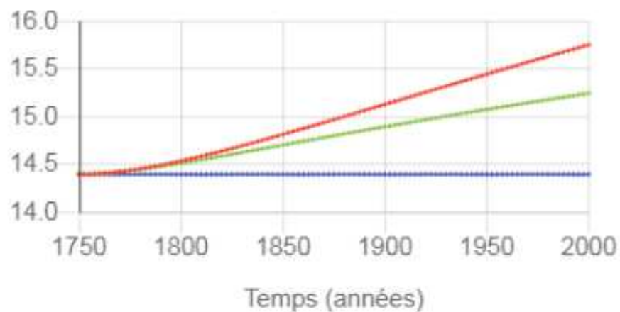
Figure 11: Copie d'écran des résultats d'une simulation pré-industrielle avec concentration en \text{CO}_2 constante (bleu) et avec des émissions anthropiques qui permettent de faire passer la concentration en \text{CO}_2 à la concentration actuelle (rouge). La simulation verte est identique à la rouge, sauf que la rétro-action de la vapeur d'eau a été débranchée en maintenant constante la concentration en vapeur d'eau. Notons que pour la concentration en \text{CO}_2 , la courbe verte se trouve cachée par la courbe rouge.
