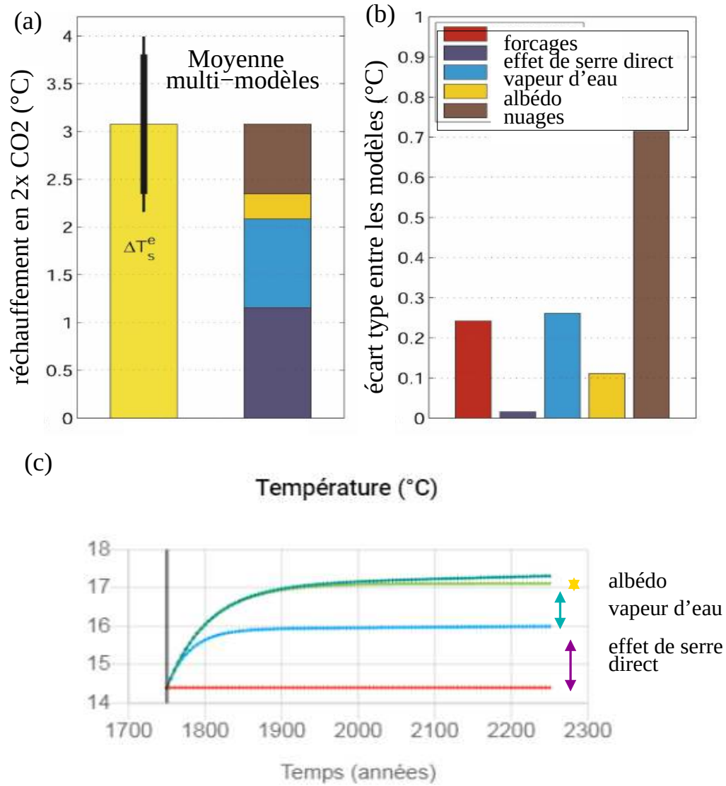
Figure 17: Comparaison des rétroactions climatiques lors d'un doublement de CO_2 produites par SimClimat et par les modèles de climat participant à CMIP. (a) Réchauffement climatique et ses contributions simulés par la moyenne des modèles de climat. (b) Écart type des différentes contributions au réchauffement simulées par les différents modèles de climat. (c) Évolution de la température simulée par SimClimat, avec et sans les différentes rétroactions. La courbe rouge est une simulation pré-industrielle, la courbe vert foncé est une simulation avec CO_2 doublé (560 ppm), la courbe vert clair est une simulation avec CO_2 doublé et albédo constant, et la courbe bleue est une simulation avec CO_2 doublé et concentration en vapeur d'eau constante. Les panels (a) et (b) sont issus de [Dufresne and Bony, 2008].
