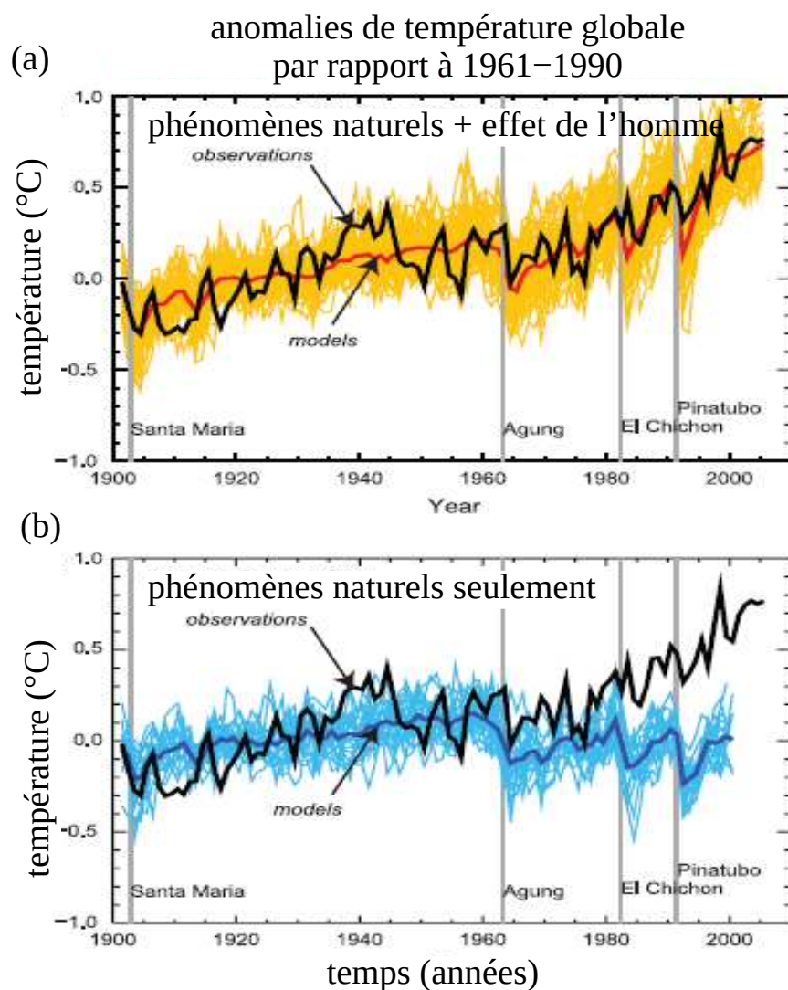
Figure 18: (a) Évolution de la température globale depuis 1900 pour les observations (noir), pour les modèles participant à CMIP (jaune) et pour la moyenne entre tous les modèles de CMIP (rouge), lorsque la concentration en gaz à effet de serre augmente de la même manière que dans les observations. (b) Évolution de la température globale depuis 1900 pour les observations (noir), pour les modèles participant à CMIP (bleu clair) et pour la moyenne entre tous les modèles de CMIP (bleu foncé), lorsque la concentration en gaz à effet de serre reste constante. Figure issue du 5e rapport du GIEC ([ IPCC, 2013 ]).
