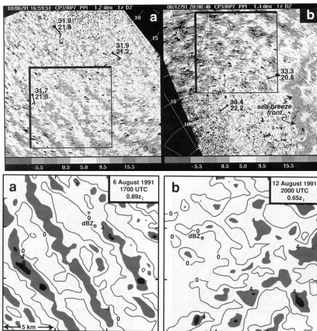
FIG. 13 – En haut, champs de réflectivité radar pour 2 situations particulières observées en Floride (a) le 6 août 1991 à 1700 UTC et (b) le 12 août 1991 à 2000 UTC. La température (nombre du haut) et le point de rosée (nombre du bas) ainsi que le vent sont superposés pour certaines stations d'observation. La figure de gauche montre une couche limite régulièrement organisée en rouleaux. La figure de droite montre un front de brise de mer sur la droite et des cellules en haut. Les figures du dessous correspondent à un lissage des échos radar pour le sous-domaine repéré par un carré dans les figures du haut, avec des contours tous les 4 dBZ e à partir de 0. Les valeurs plus grandes que 4 et 8 dBZ e sont grisées respectivement en gris clair et gris foncé. D'après Weckwerth et al. (1997).
