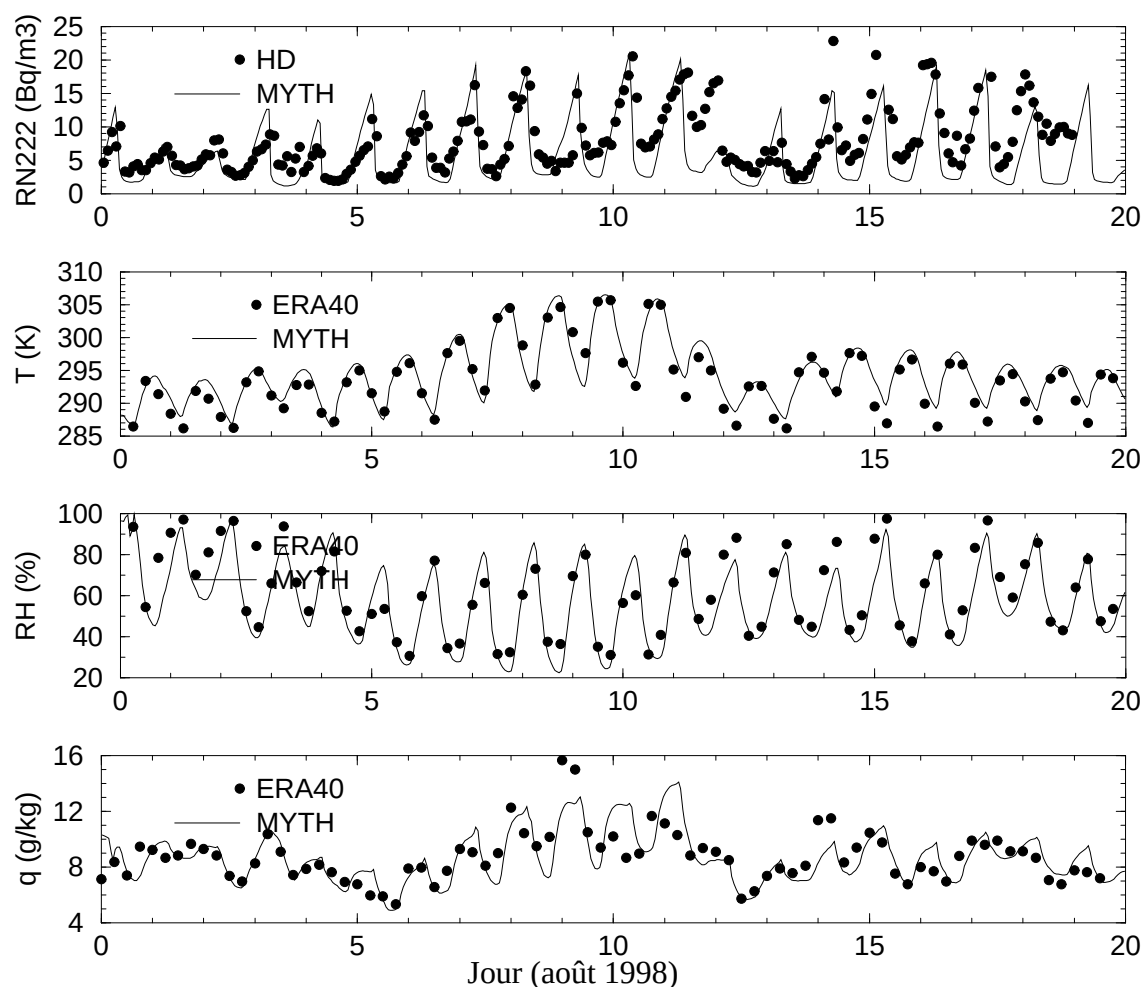
FIG. 24 – Evolution, pour la période du 1 au 20 août 1998, de la concentration de radon en surface à Heidelberg (en haut, \text{Bq m}^{-3} ), et, dans la première couche du modèle, de la température (K), de l'humidité relative (%) et de l'humidité spécifique (g/kg). Pour les trois courbes du bas, les données correspondent aux réanalyses ERA40 interpolées dans la couche correspondante.
