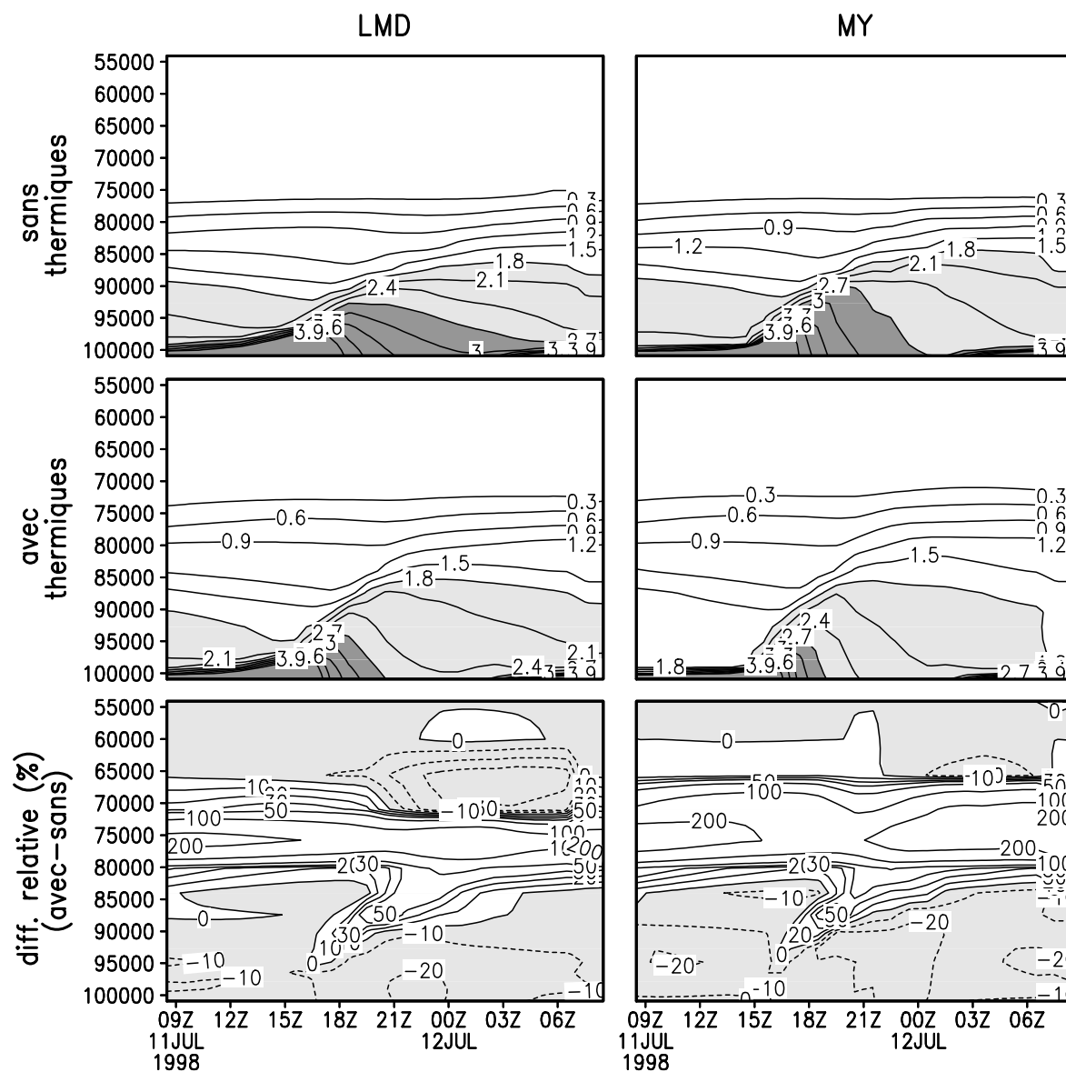
FIG. 28 – Cycle diurne moyen (du 7 au 10 août 1998) du profil vertical (axe des ordonnées en Pa) de radon ( \text{Bq m}^{-3} ) simulé à Heidelberg avec pour la diffusion turbulente, soit la paramétrisation LMD(+CG) (à gauche) soit la paramétrisation MY (à droite). On montre les simulations sans (en haut) et avec (en bas) thermiques ainsi que la différence relative entre les deux (avec moins sans).
