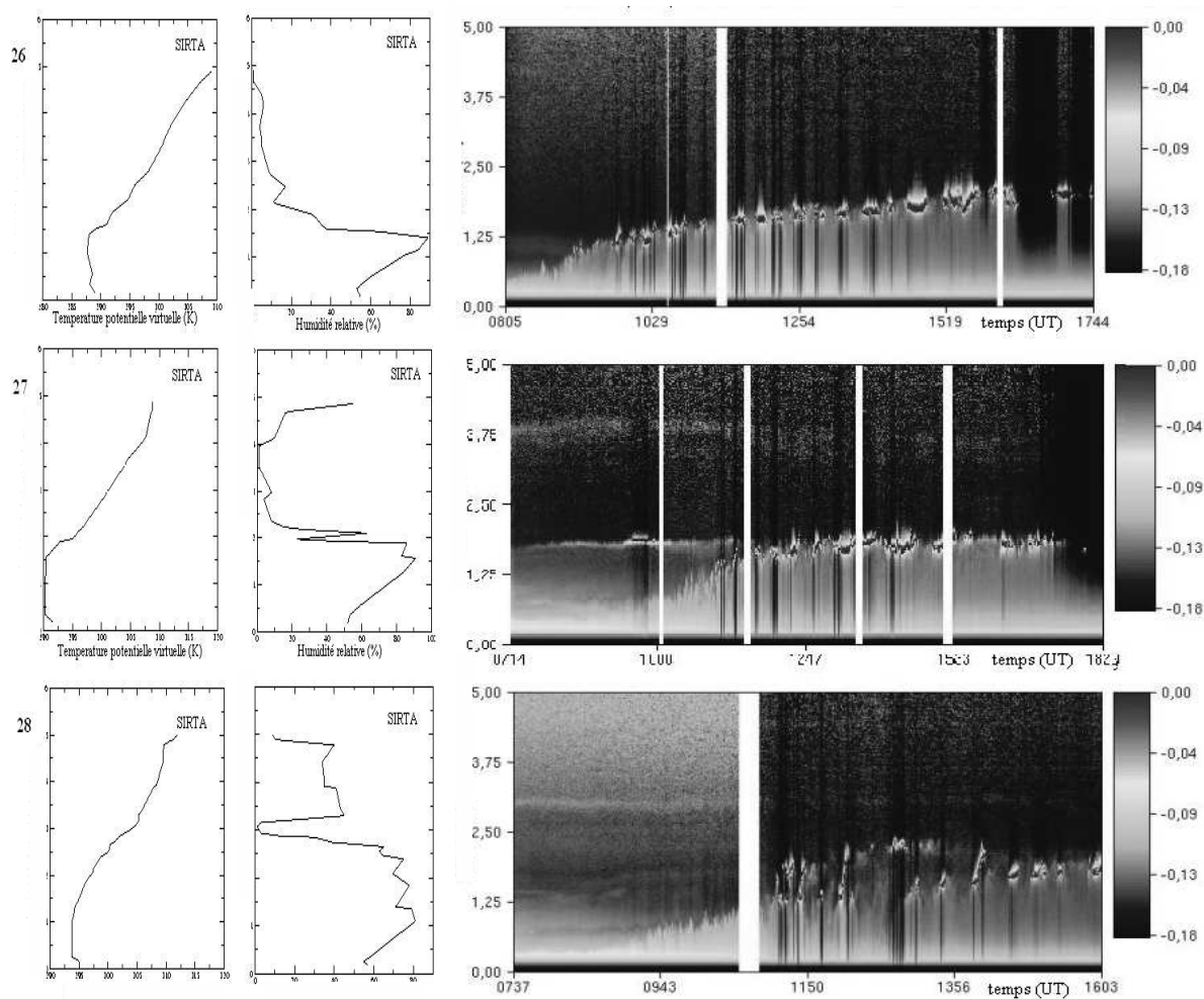
FIG. 14 – Cycle diurne de la couche limite continentale.
