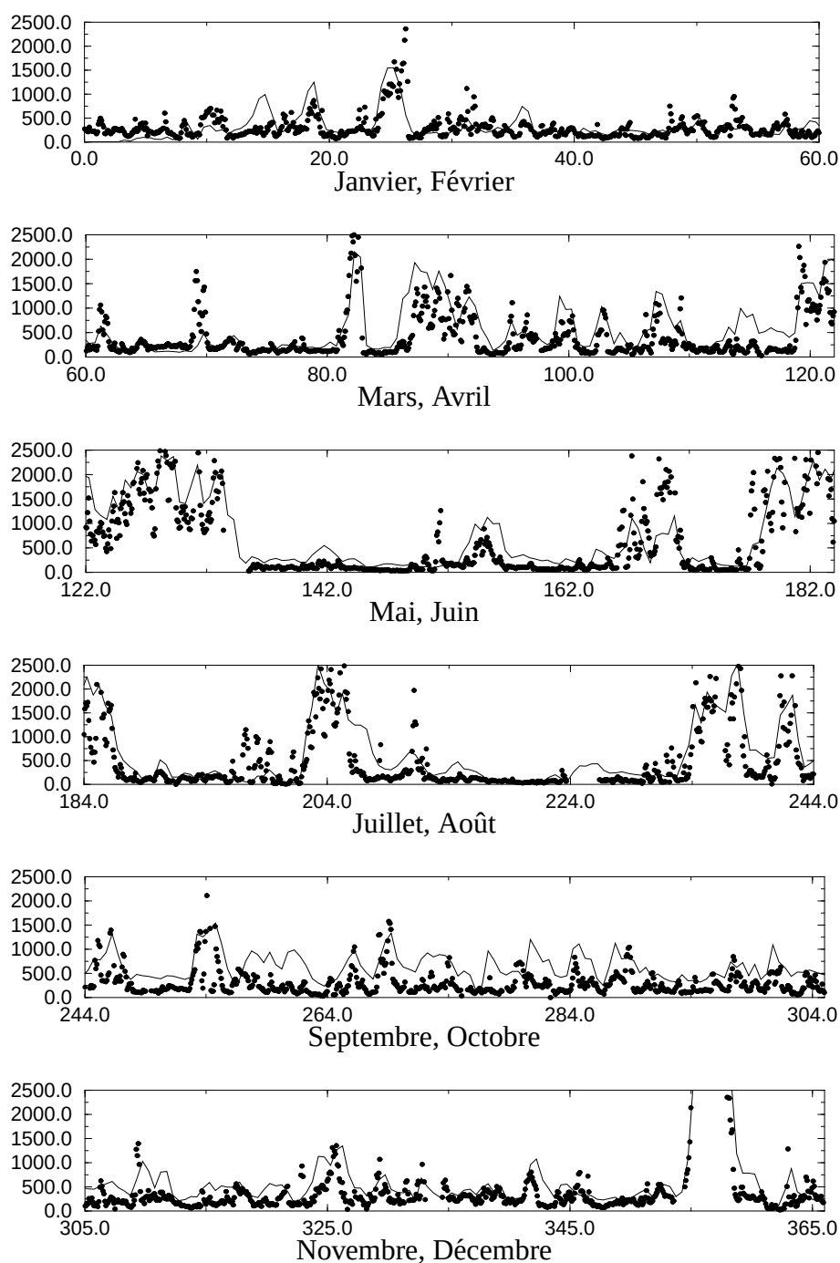
FIG. 33 – Mesure (points) et simulation (trait) du ^{222}\text{Rn} ( \text{mBq/m}^3 ) à Mace Head pour l'année 2000. La simulation est réalisée avec le modèle LMDZT guidé par les analyses ECMWF en utilisant une grille régulière avec une résolution de 2^\circ \times 2^\circ .
