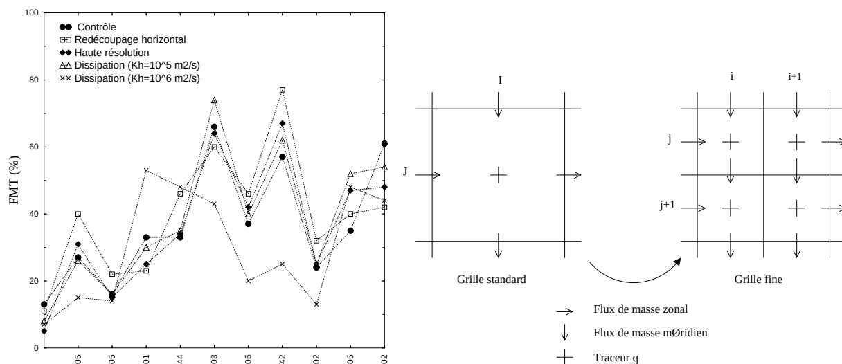
FIG. 37 – Sensibilité des simulations ETEX à la résolution horizontale et à la dissipation. La simulation de contrôle a une maille de 120 km de côté. On teste des grilles deux fois plus fines dans les deux directions. La simulation “Haute résolution” correspond à un cas où on recalcule la météorologie et le transport sur une grille plus fine. Dans la simulation avec “Redécoupage horizontal”, on utilise les archives de la simulation de contrôle mais on redécoupe la maille horizontalement pour le transport suivant le schéma de droite. Cette solution permet de diminuer la diffusivité sans avoir à recalculer la météorologie. Ses résultats sont très proches de ceux de la simulation “Haute résolution”. On teste également l’impact d’introduire une dissipation horizontale avec pour coefficient de dissipation K_h , 10^5 ou 10^6 \text{ m}^2 \text{ s}^{-1} .
