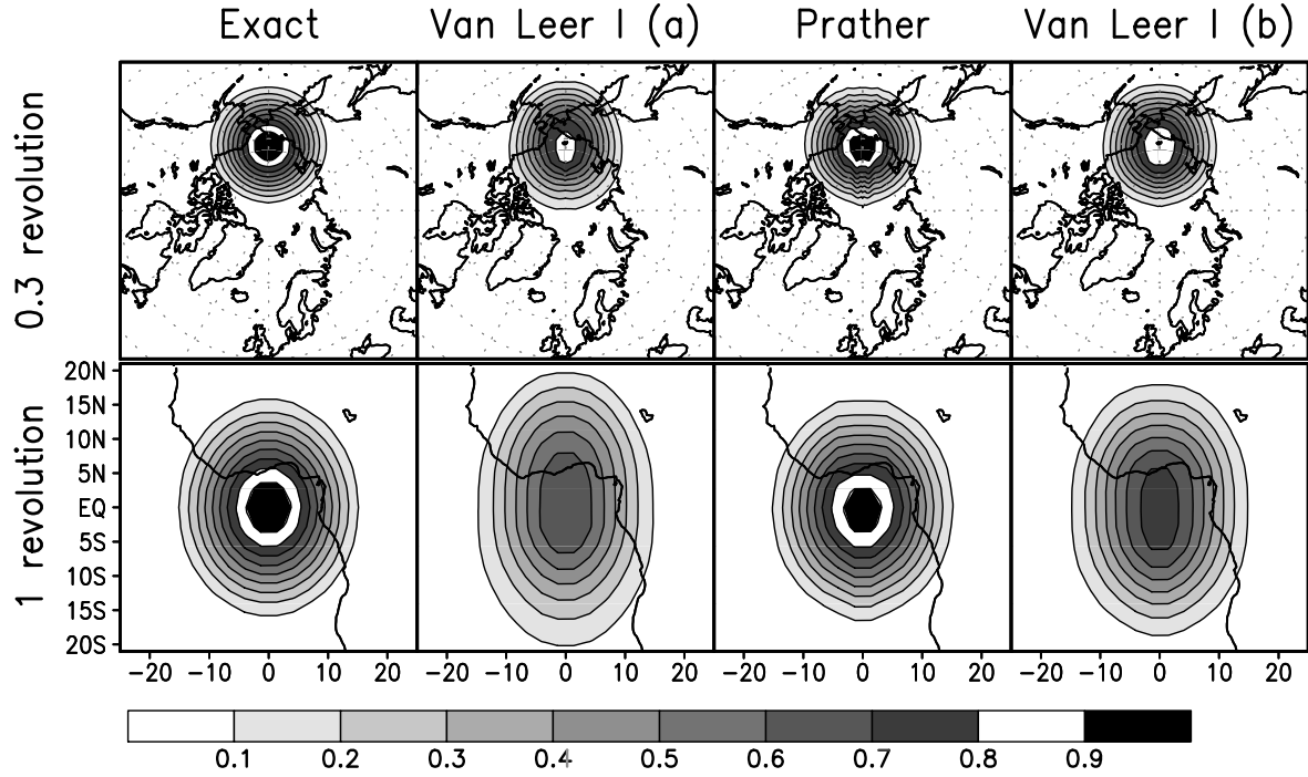
FIG. 5 – Test numérique d’advection transpolaire. Suivant Williamson et Rasch (1989) et Allen et al. (1991), la distribution initiale de traceur est donnée par c(\lambda, \phi) = (1 + \cos[\min(r[\lambda, \phi]/R, 1)])/2 avec r = \arccos(\cos \lambda \cos \phi) et R = 7 \times (2\pi)/128 . La grille utilisée comprend 128 points en longitude et 64 en latitude. On montre de gauche à droite, la solution exacte, un test du schéma I de Van Leer avec 16000 pas de temps (pour avoir un nombre de Courant plus petit que 1) pour une révolution complète, un test du schéma de Prather avec le même pas de temps et enfin une simulation avec le schéma I mais seulement 160 pas de temps. Les graphiques du haut montrent la distribution de traceur juste après le premier passage par un pôle. Les graphiques du bas montrent le résultat obtenu après une révolution complète autour du globe.
