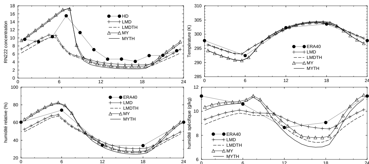
FIG. 25 – Cycle diurne moyen du radon en surface à Heidelberg et, dans la première couche du modèle, de la température, de l'humidité relative et spécifique dans la première couche du modèle (période du 7 au 10 août).
