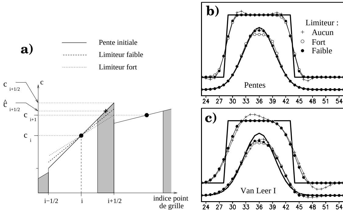
FIG. 3 – a) Illustration de l'application d'un limiteur de pente. A droite, impact des limiteurs de pentes sur le schéma des pentes ( b ) et sur le schéma I de Van Leer ( c ). Les cas sans limiteurs (les mêmes que sur la Fig. 2) et les limiteurs faibles et forts (se reporter au texte pour plus de détails) sont montrés pour les distributions carrée et gaussienne.
