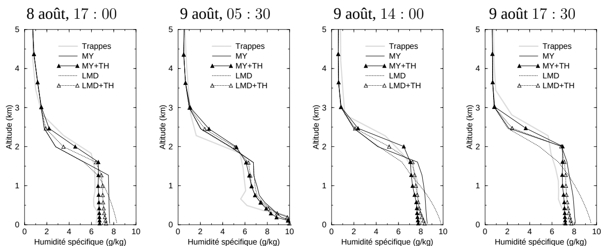
FIG. 30 – Profils d’humidité spécifique simulés et observés à Trappes.
