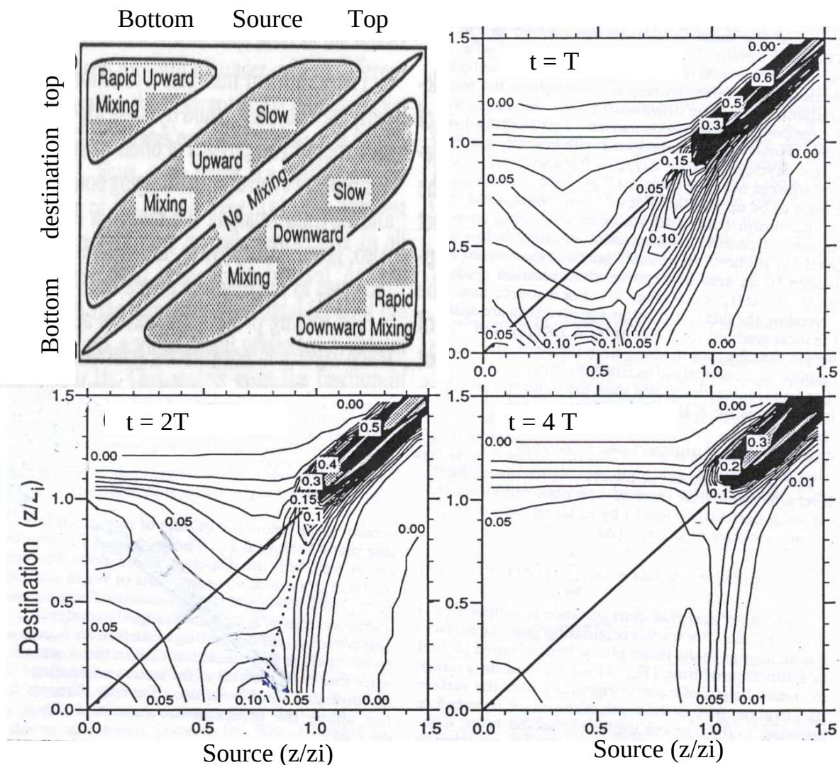
FIG. 20 – Calcul et interprétation d’une matrice de transience à partir d’une simulation des grands tourbillons dans une couche limite convective. D’après Ebert et al. (1989).
