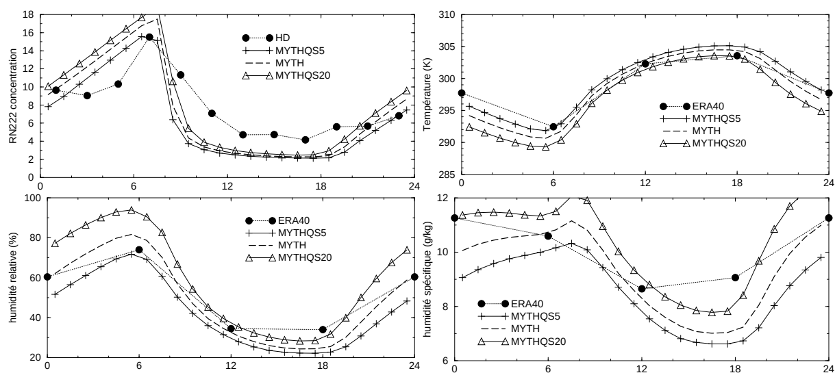
FIG. 27 – Influence de l'humidité du sol. Cycles diurnes du radon, de l'humidité et de la température (période du 7 au 10 août 1998) pour la simulation nominale (MYTH, contenu en eau du sol de 10 mm) et des simulations avec un contenu divisé (MYTHQS5) ou multiplié (MYTHQS20) par 2.
