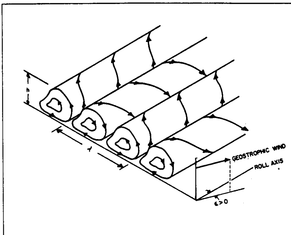
FIG. 10 – Vue schématique de l'organisation de la convection de couche limite en rouleaux, le long de l'axe du vent. D'après Brown (1980).
