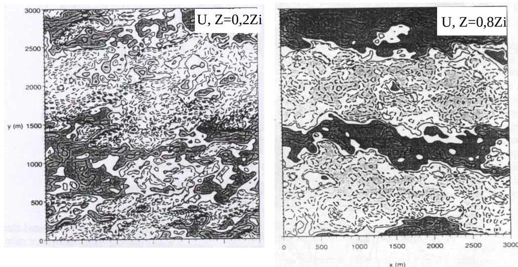
FIG. 12 – Perturbation du vent zonal à deux altitudes dans la simulation SB1 de Moeng et Sullivan (1994).
