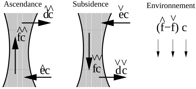
FIG. 7 – Notations pour le transport en flux de masse des traceurs par la convection.
