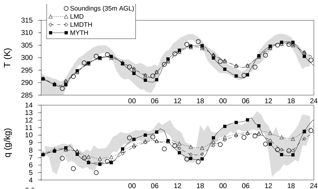
FIG. 26 – Evolution de la température et de l'humidité spécifique à Trappes et pour trois des simulations pour les 7, 8 et 9 août, journées pour lesquelles on dispose des radiosondages à haute fréquence. Les valeurs simulées correspondent à la première couche du modèle et sont donc à comparer aux données de Trappes à 35 m.
