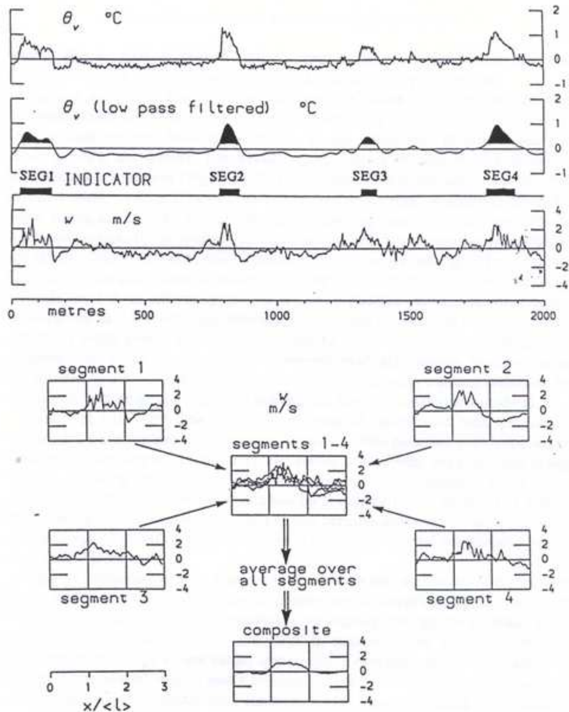
FIG. 16 – Principe d’une analyse en composites d’évènements chauds de mesures avions de la turbulence de couche limite. La partie du haut montre une séquence de mesures de la température potentielle et du vent vertical. Une courbe lissée des températures potentielles est utilisée pour identifier les évènements chauds. Chaque évènement est associé à un segment qui est ensuite étiré dans l’espace pour ramener tous les segments à une longueur identique. Pour chaque variable, on peut alors construire des moyennes ou des écart-types pour un thermique moyen. La figure et l’approche sont issues d’une très jolie étude de Williams et Hacker (1992).
