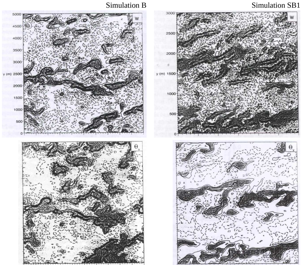
FIG. 11 – Simulations des grands tourbillons de la couche limite convective d'après Moeng et Sullivan (1994). Coupes horizontales instantanées à 0, 2z_i pour deux simulations (B à gauche et SB1 à droite). On montre, en haut, le vent vertical w ( \text{m s}^{-1} ) et, en bas, les perturbations de température potentielle virtuelle \theta'_v (K).
