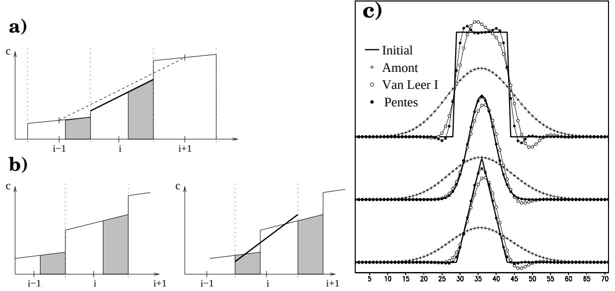
FIG. 2 – Schémas du 2nd ordre. Illustration de l'estimation de la pente par différences finies pour le schéma I de Van Leer (a) et par calcul par moindres carrés à partir de la distribution en ligne brisée résultant de l'advection au pas précédent (b). Cette seconde estimation correspond au schéma des pentes de Russell et Lerner (1981) ou au schéma III de Van Leer (se reporter au texte pour plus de détails). c : Exemples de calculs d'advection unidimensionnelle sur un domaine périodique de 70 points (axe horizontal), avec une vitesse constante u et trois distributions initiales. Les concentrations de traceur ( c , unité arbitraire) sont montrées après une révolution complète, au pas de temps 350 pour un nombre de Courant U/m = 0, 2 .
