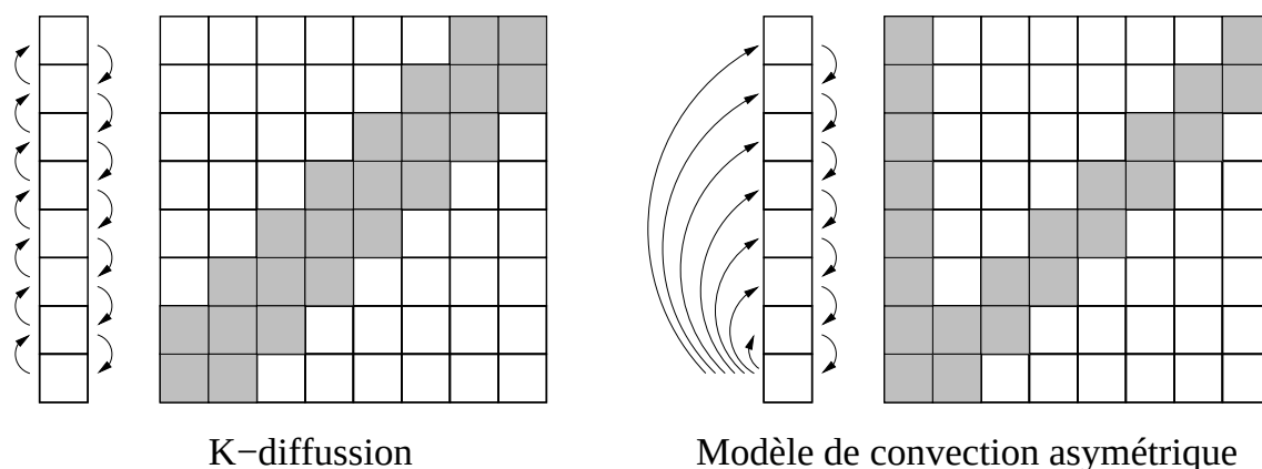
FIG. 21 – Forme prise par les matrices de transilience (ou d'échange) dans le cas d'une formule en diffusion turbulente à gauche et dans le cas du modèle de convection asymétrique de Pleim et Chang (1992) à droite. On montre par des flèches sur des colonnes verticales les échanges mis en jeu dans ces paramétrisations et en grisé les éléments non nuls de la matrice associée.
