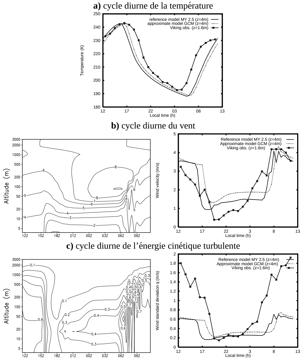
FIG. 8 – Cycle diurne de la couche limite sur Mars. Comparaison d'observations par les sondes Viking (qui ont fonctionné plusieurs années à la surface de Mars dans les années 70) et les résultats de simulations numériques effectuées avec une version unidimensionnelle du modèle de circulation générale martien du LMD. a : Cycle diurne de la température de l'air mesurée au bout du bras Viking (à 1,6 m au-dessus du sol) et simulée dans la première couche du modèle (altitude de 4 m). b : Module du vent horizontal ( \text{m s}^{-1} ). c : Fluctuations turbulentes du vent ( \text{m s}^{-1} ). Pour b) et c), on montre, à gauche , les résultats du modèle en fonction de l'heure locale et de l'altitude et, à droite , les évolutions comparées des mêmes grandeurs près de la surface pour le modèle et les observations Viking. Les axes horizontaux correspondent aux heures locales. Pour les fluctuations turbulentes (c), les données sont calculées à partir de mesures haute fréquence du vent et les valeurs simulées sont estimées à partir de l'énergie cinétique turbulente prédite par la paramétrisation de Mellor et Yamada.
