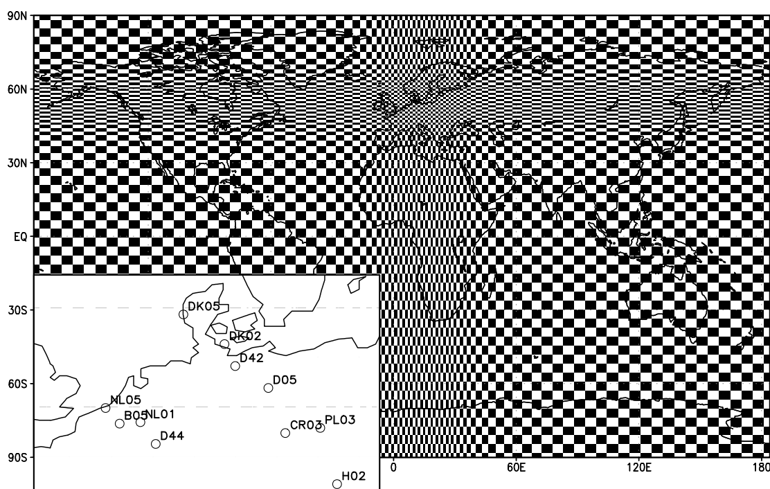
FIG. 34 – Grille retenue pour les simulations ETEX-1 et localisation des 11 stations retenues pour les diagnostics d'intercomparaison.
