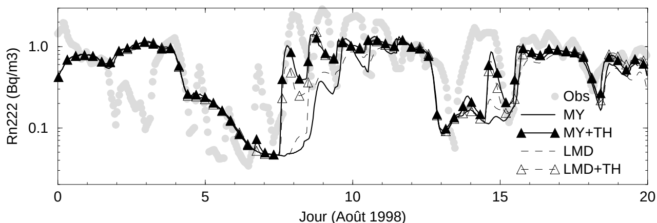
FIG. 29 – Evolution sur le mois d’août 1998 de la concentration de radon observée à la station Jungfraujoch, située à 3400 m d’altitude, et simulée au même point et dans la couche du modèle située à cette même altitude.
