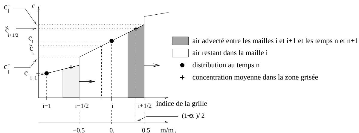
FIG. 1 – Principe du schéma de Van Leer et notations. On montre le cas où la distribution sous-maille est représentée au moyen d'un polynôme du premier degré. L'axe vertical correspond à la concentration massique du traceur. Les deux axes horizontaux correspondent à l'indijage des variables et à la masse d'air comptée à partir du centre de la maille i et normalisée par la masse totale de cette même maille, m_i . La surface grisée correspond à la quantité de traceur qui est transféré au travers de l'interface durant un pas de temps.
