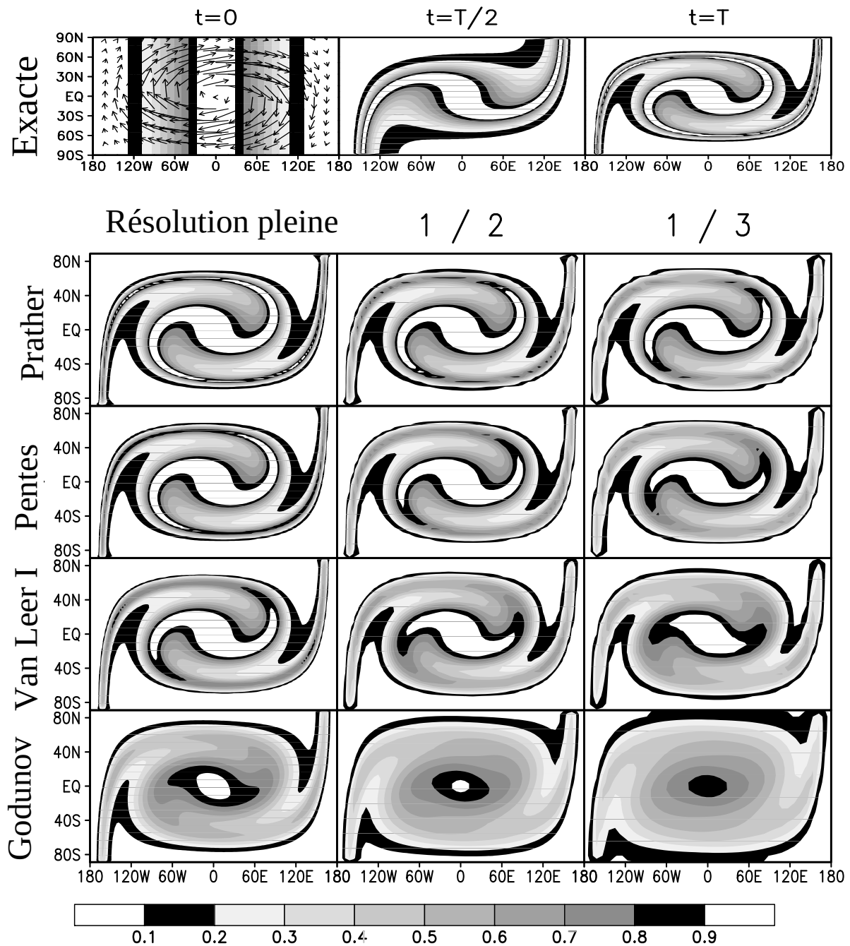
FIG. 6 – Tests d'advection bidimensionnelle avec un champ de vent analytique. La distribution initiale de traceur est une fonction gaussienne de la longitude. Les graphiques du haut montrent l'état initial (à gauche) et la solution exacte aux instants T/2 et T . Le temps T correspond à une révolution complète au centre du domaine. En dessous, on montre les résultats numériques au temps T pour différents schémas d'advection et 3 résolutions : résolution pleine, 1/2 et 1/3, correspondant respectivement à des grilles longitude-latitude de 120 \times 60 , 60 \times 30 et 40 \times 20 points.
