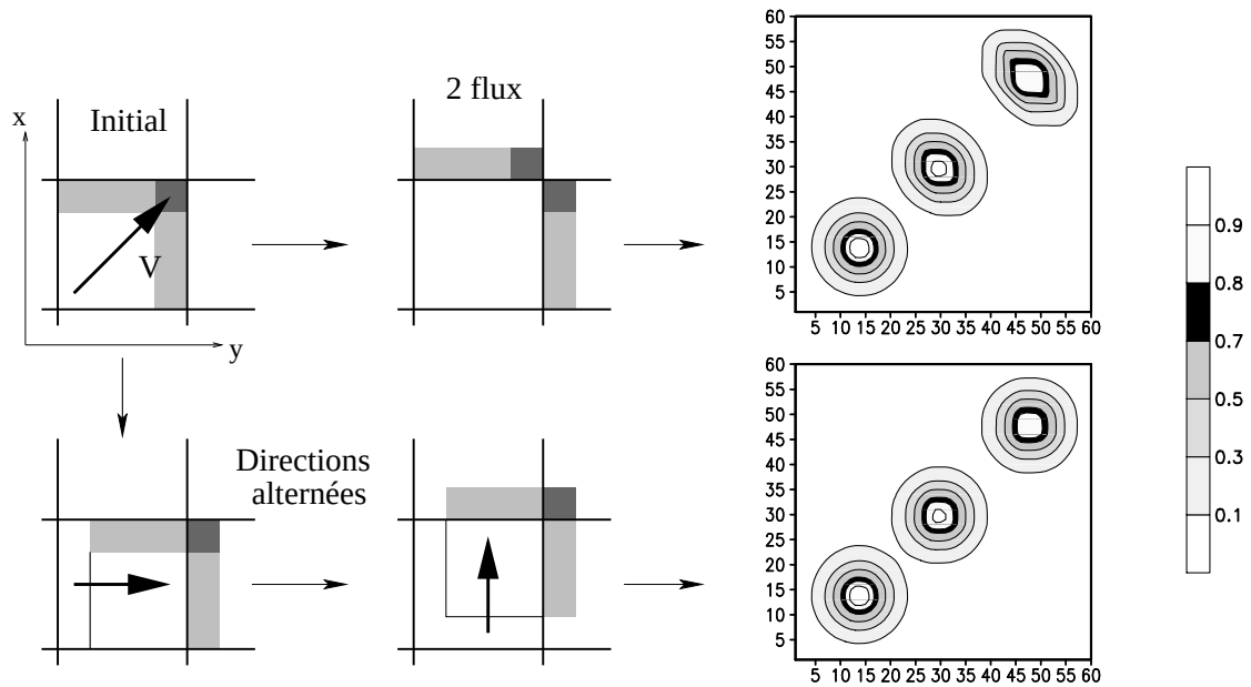
FIG. 4 – Advection uniforme d'un pic gaussien de concentration le long de la diagonale d'un maillage bidimensionnel régulier. En haut, le calcul de la divergence des flux est effectué à partir de flux estimés indépendamment en x et en y . La ligne du bas montre un calcul alterné avec d'abord une advection en x puis une advection en y . Ces illustrations numériques ont été réalisées avec le schéma I de Van Leer, sur un maillage de 60 points dans chaque direction horizontale.
