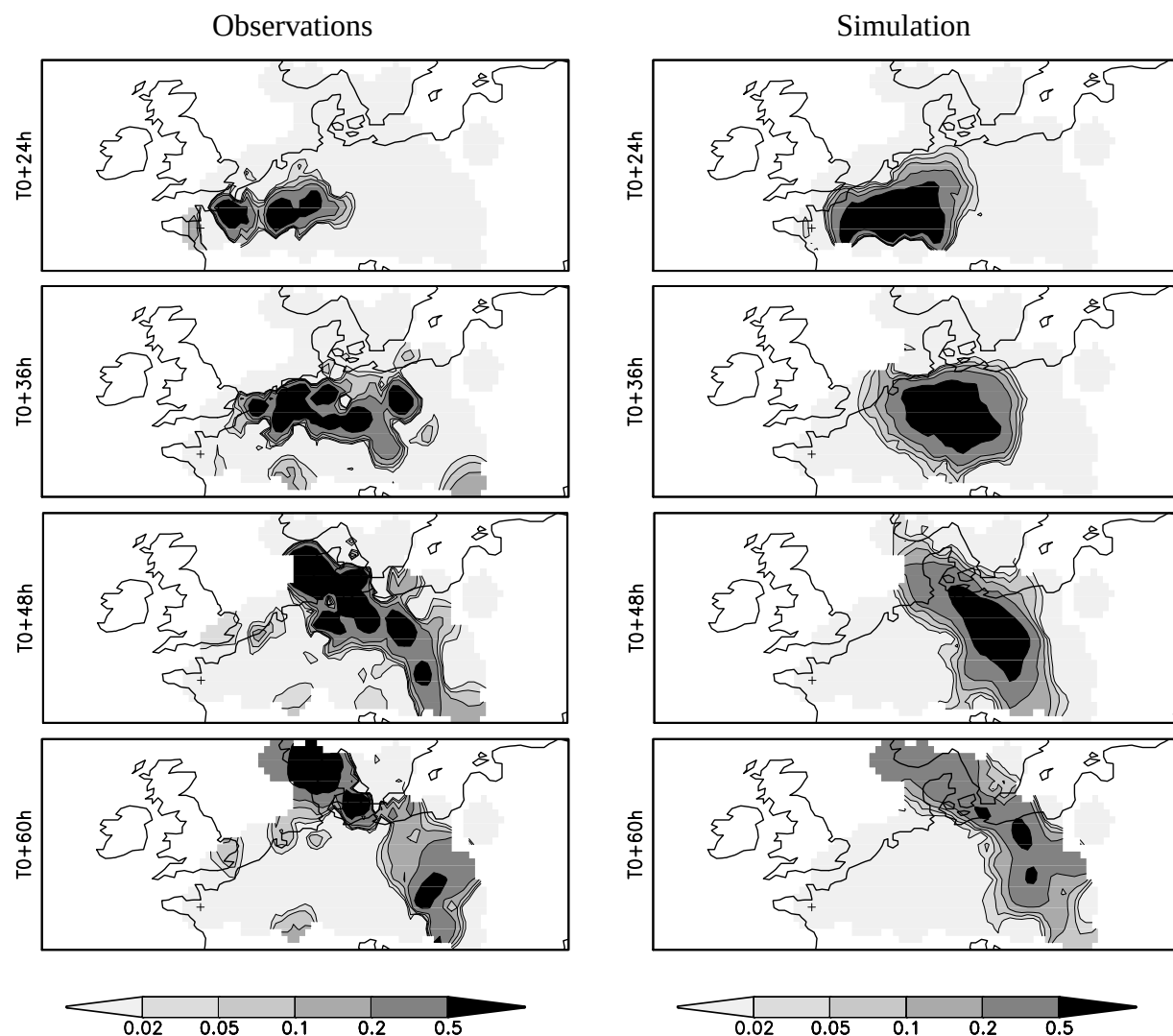
FIG. 35 – Panaches de PMCH ( \text{ng m}^{-3} ) observés et simulés pour la campagne ETEX. Le panache est reconstitué à partir des mesures aux stations en appliquant un filtre de Cressman (1959) utilisable depuis le logiciel graphique du domaine public GrADS utilisé pour ces figures. Les concentrations sont en ng par kg d'air. Les heures sont comptées par rapport au temps T0 de relâchage du PMCH. Pour la simulation, plutôt que de tracer le panache directement, on commence par extraire pour chacune des 168 stations la séquence des concentrations simulées (en prenant la valeur au point de grille le plus proche) puis on reconstitue le panache avec la même méthode que pour les observations.
