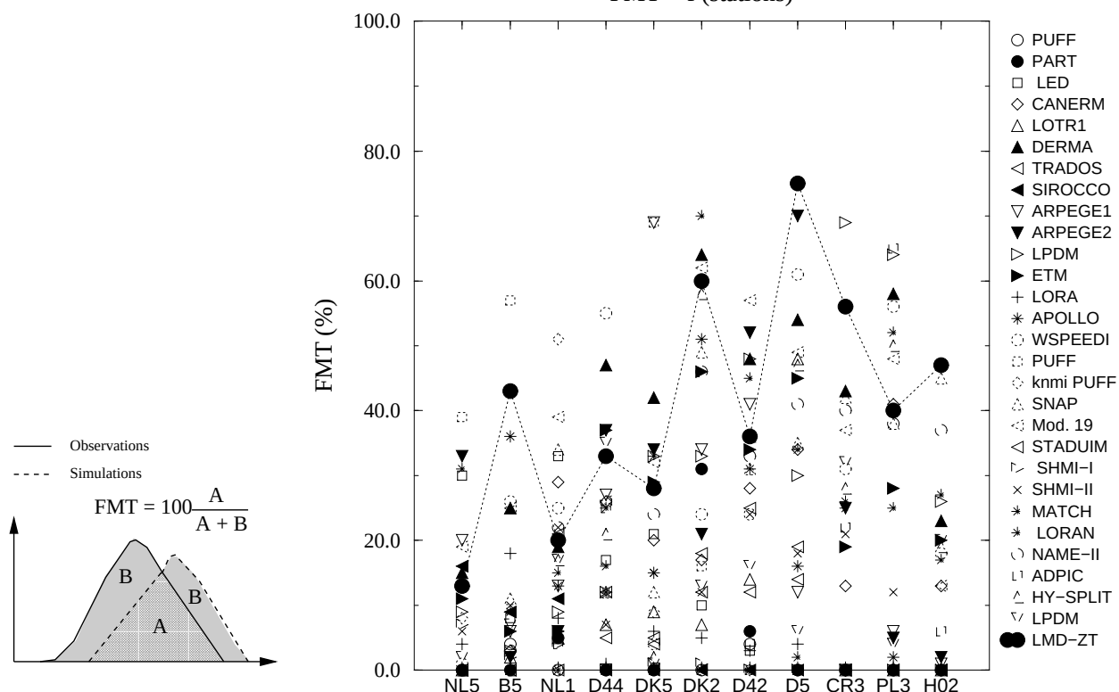
FIG. 36 – Schéma illustrant le critère FMT (à gauche) et FMTs calculés pour les 11 stations de la Fig. 34 et pour un grand nombre de modèles utilisés dans le cadre d'ETEX et pour LMD-ZT (à droite).
