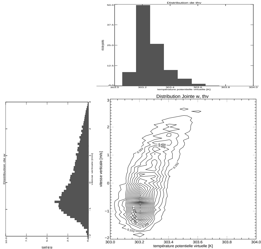
FIG. 18 – Distributions et distributions croisées des vitesses verticales et des fluctuations de la température potentielle virtuelle dans des simulations des grands tourbillons effectuées avec le modèle mésoNH pour un cas de couche limite convective observé dans les grandes plaines américaines pendant la campagne IHOP le 14 juin 2002. Des observations radar de ce cas particulier sont présentées sur la Fig. 15.
