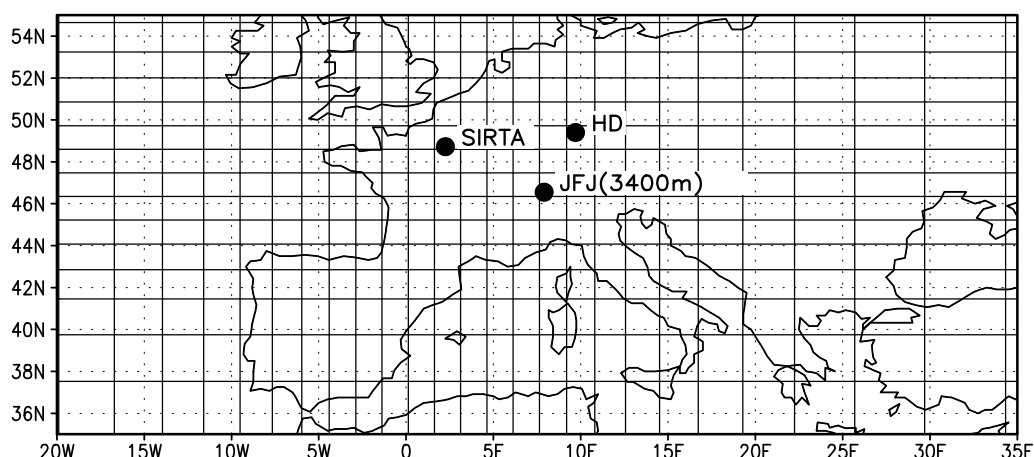
FIG. 23 – Grille utilisée pour les simulations guidées et zoomées sur la France avec l’emplacement du Sirta et des stations radon de HD et JFJ.
