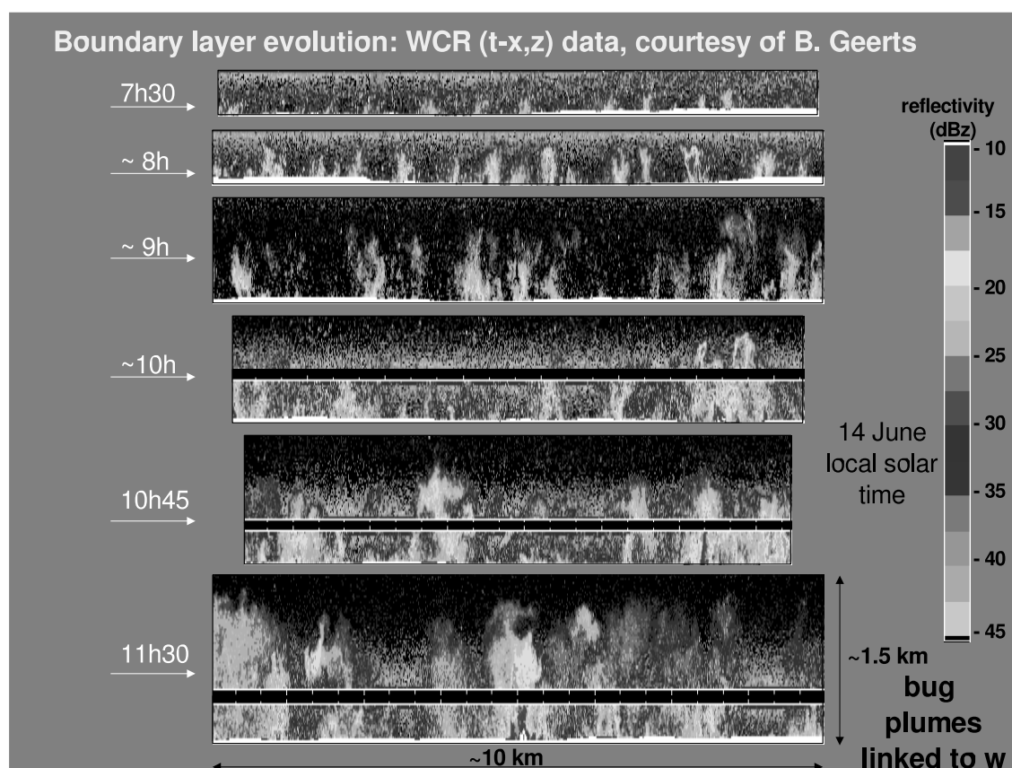
FIG. 15 – Observations de la couche limite en Oklahoma le 14 juin 2002 pendant la campagne IHOP. Transects avions à différentes heures de la journée avec des mesures radar en dessous et au-dessus de l’avion. On voit bien la croissance des thermiques qui atteignent, en milieu de journée, environ 1,5 km.
