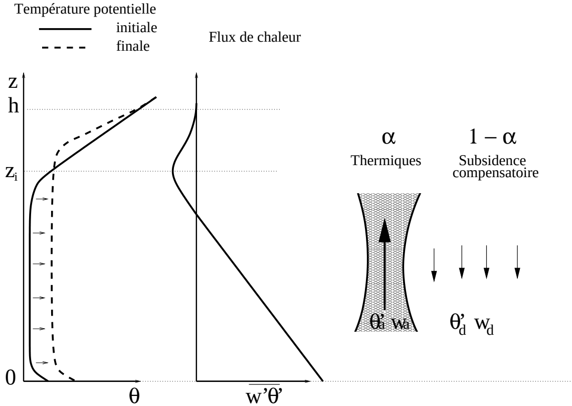
FIG. 19 – Représentation schématique de la couche limite convective
