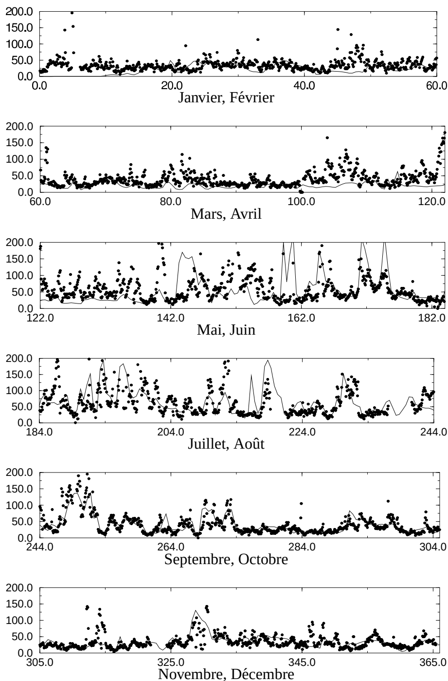
FIG. 32 – Mesure (points) et simulation (trait) du ^{222}\text{Rn} ( \text{mBq/m}^3 ) à l'île d'Amsterdam pour l'année 2000. La simulation est réalisée avec le modèle LMDZT guidé par les analyses ECMWF en utilisant une grille régulière avec une résolution de 2^\circ \times 2^\circ .
