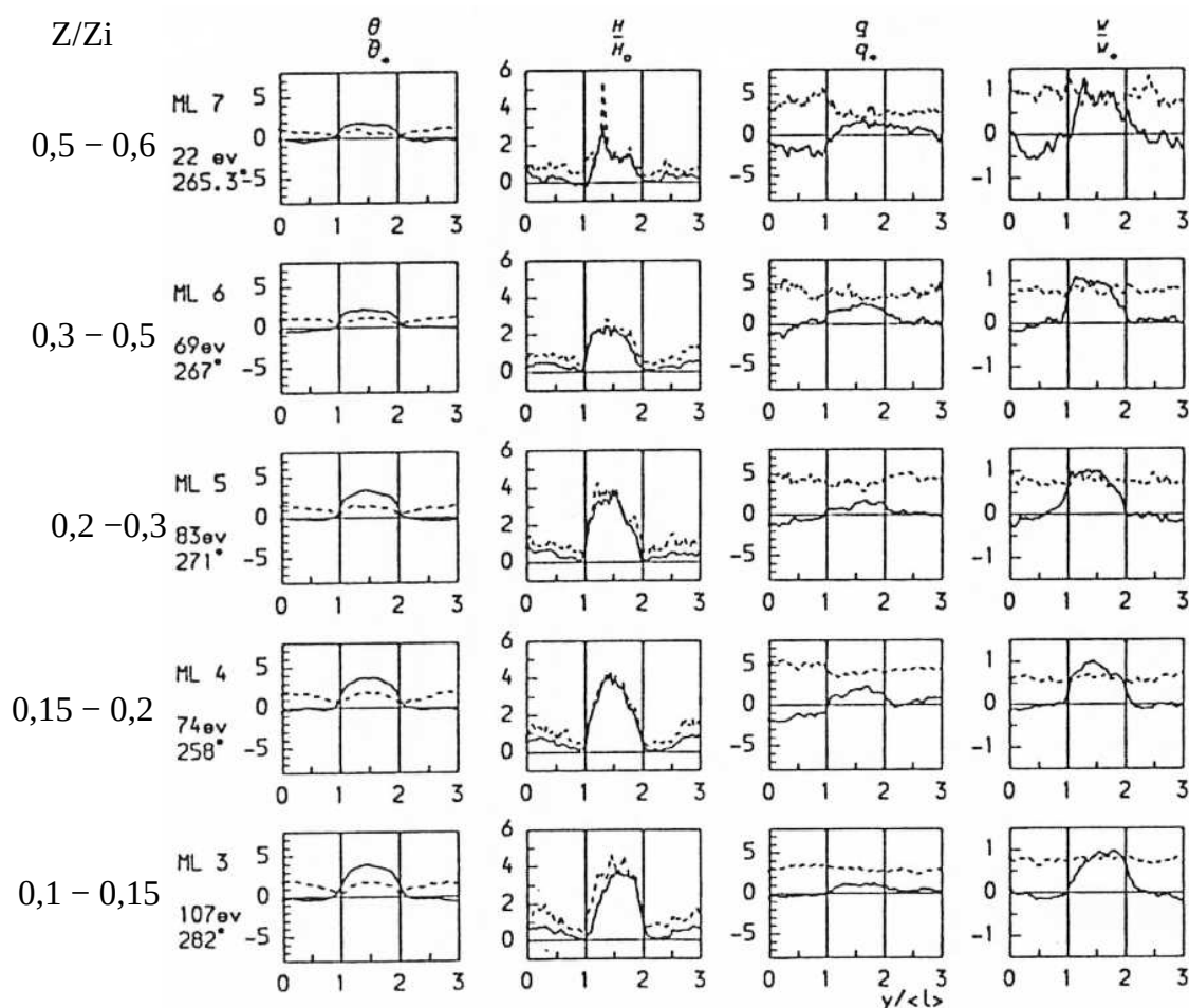
FIG. 17 – Analyse en composites d'évènements chauds d'une série de vols avion effectués dans la couche limite convective en Australie. Les rangées correspondent à différentes gammes de valeurs de z/z_i . Les deux rangées du haut correspondent au milieu de la couche mélangée. De gauche à droite sont représentés, la température potentielle \theta , le flux de chaleur H = \rho C_p \overline{w'\theta'} , l'humidité spécifique q et la vitesse verticale w , normalisées par les échelles \theta^* , H_0 = \rho C_p \overline{w'\theta'_0} , q^* et w^* . Les courbes pleines correspondent aux moyennes des grandeurs et les courbes pointillées aux écart-types associés. Le nombre d'évènements associés à chaque mesure est donné à gauche (22ev par exemple veut dire qu'on a fait des statistiques avec 22 segments). D'après Williams et Hacker (1992).
