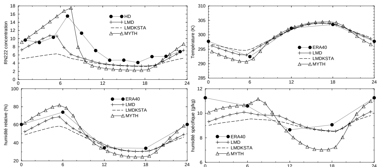
FIG. 31 – Influence de la paramétrisation de la couche de surface. Cycles diurnes du radon, de l'humidité et de la température (période du 7 au 10 août 1998) pour la simulation nominale (MYTH), la simulation LMD et une simulation avec le même modèle mais avec un seuil minimum sur la diffusivité verticale introduit pour éviter les inversions trop fortes dans les régions polaires l'hiver.
