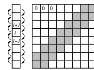
Turbulent diffusion
