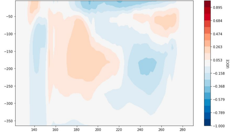
Meridional Velocity (UOCE) (DJF 1997-1998)
