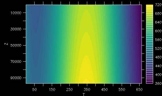
UPFLUXIR
