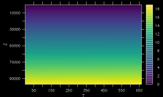
DOWNFLUXIR
