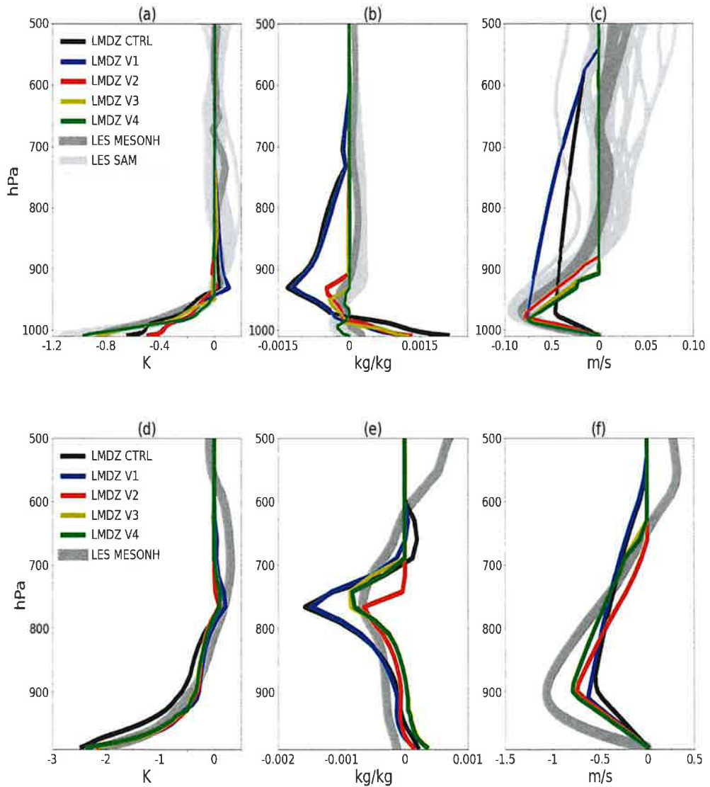
FIGURE 1.8 Profils verticaux de \delta T , \delta q et \delta w calculés dans les LES et simulés dans LMDZ contrôle (LMDZ CTRL), LMDZ avec l'ajustement du coefficient k à 0.66 (LMDZ V1), LMDZ avec la baisse de l'altitude ( h_m ) à laquelle la subsidence des masses d'air dans la poche s'annule (LMDZ V2), LMDZ avec l'ajustement de la fraction surfacique des descentes précipitantes, \sigma_{dz} , à 0.02 (LMDZ V3) et LMDZ avec l'activation des thermiques dans tout le domaine (LMDZ V4) sur le cas RCE (a, b, c) et sur le cas AMMA (d, e, f).
