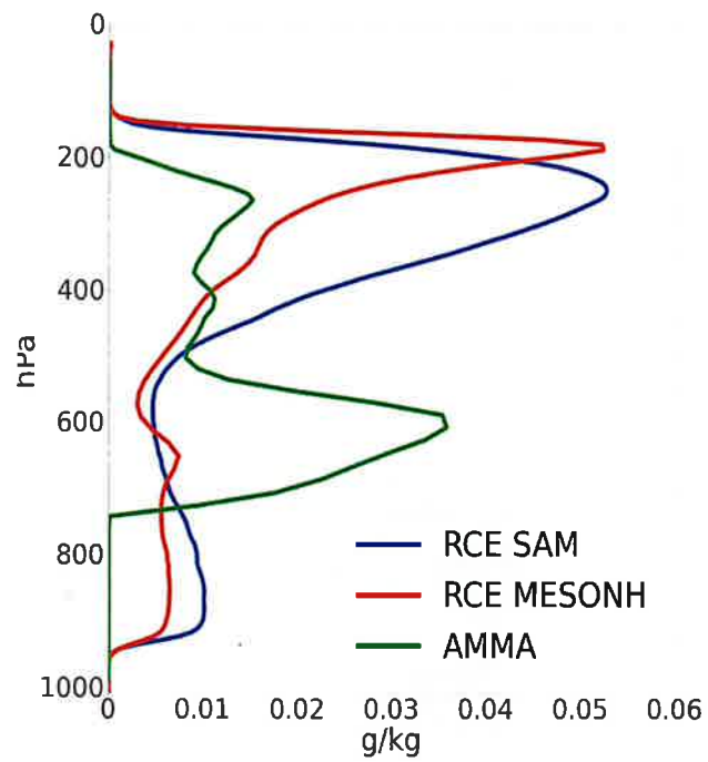
FIGURE 1.4 - Profil vertical de l'eau condensée moyennée horizontalement sur les LES en RCE océanique réalisée avec les modèles SAM et MésoNH et la LES continental du cas AMMA.
