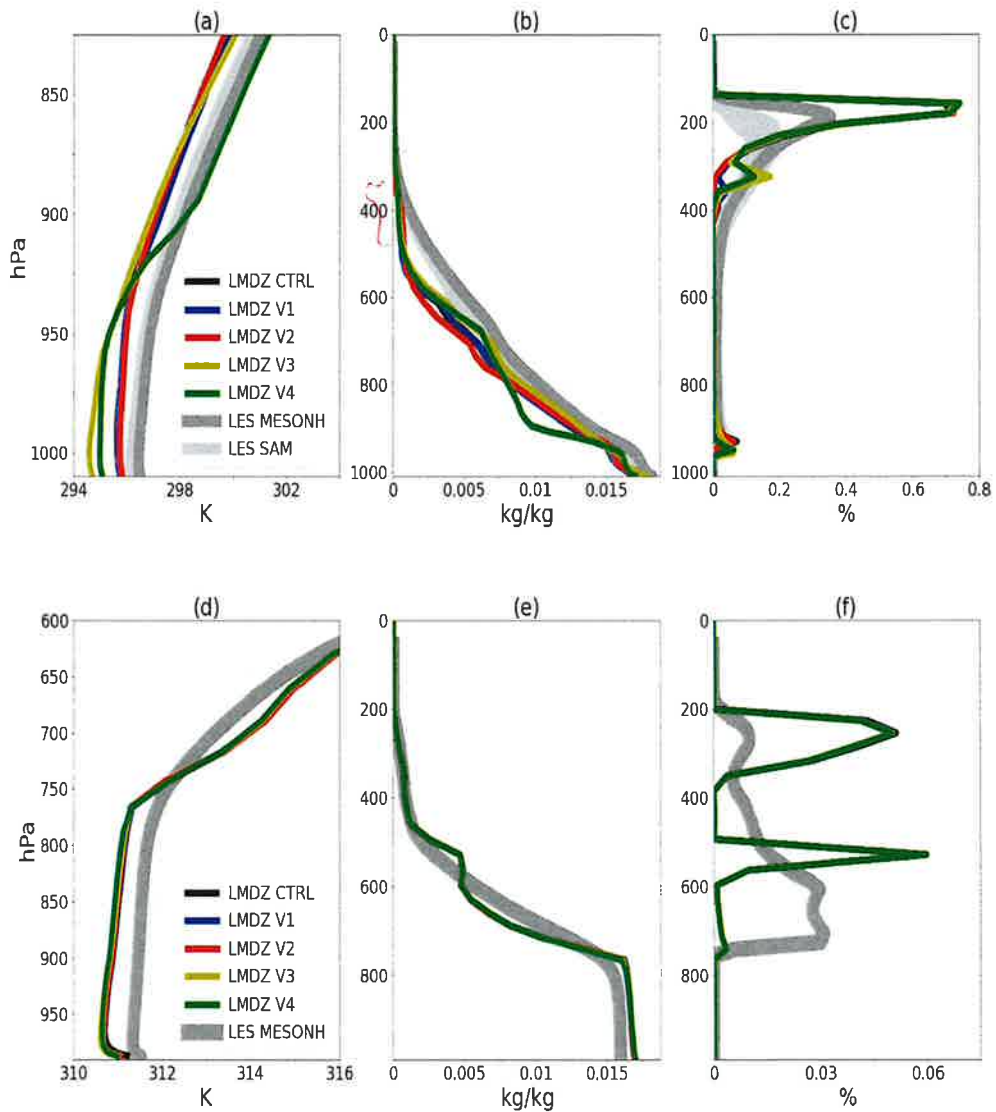
FIGURE 1.9 Profils verticaux de la température potentielle ( \theta ), de l'humidité spécifique ( qv ) et de la fraction nuageuse ( rneb ) calculés dans les LES et simulées dans LMDZ contrôle (LMDZ CTRL), LMDZ avec l'ajustement du coefficient k à 0.66 (LMDZ V1), LMDZ avec la baisse de l'altitude ( h_m ) à laquelle la subsidence des masses d'air dans la poche s'annule (LMDZ V2), LMDZ avec l'ajustement de la fraction surfacique des descentes précipitantes, \sigma_{dz} , à 0.02 (LMDZ V3) et LMDZ avec l'activation des thermiques dans tout le domaine (LMDZ V4) sur le cas RCE (a, b, c) et sur le cas AMMA (d, e, f).
