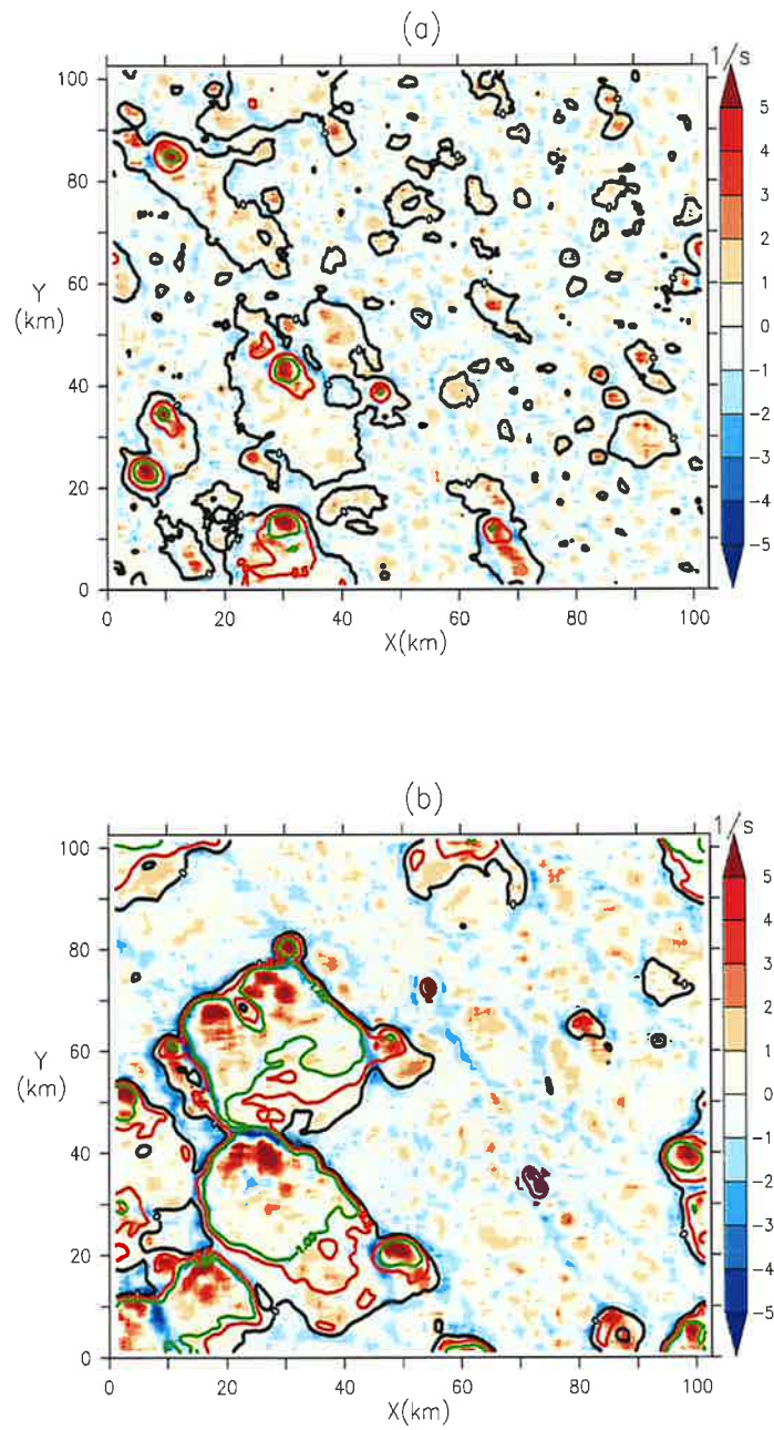
FIGURE 1.3 Carte de la divergence du vent à 10 m (en s^{-1} ) multipliée par 1000 et lissée horizontalement sur 3.25 \text{ km} \times 3.25 \text{ km} représentée sur les instants 17h10 (a) et 18h (b) de la LES MESONH réalisée sur le cas AMMA et superposés avec les contours d'anomalies de températures à 10 m à -1 K (vert), -0.5 K (rouge) et 0 K (noir)
