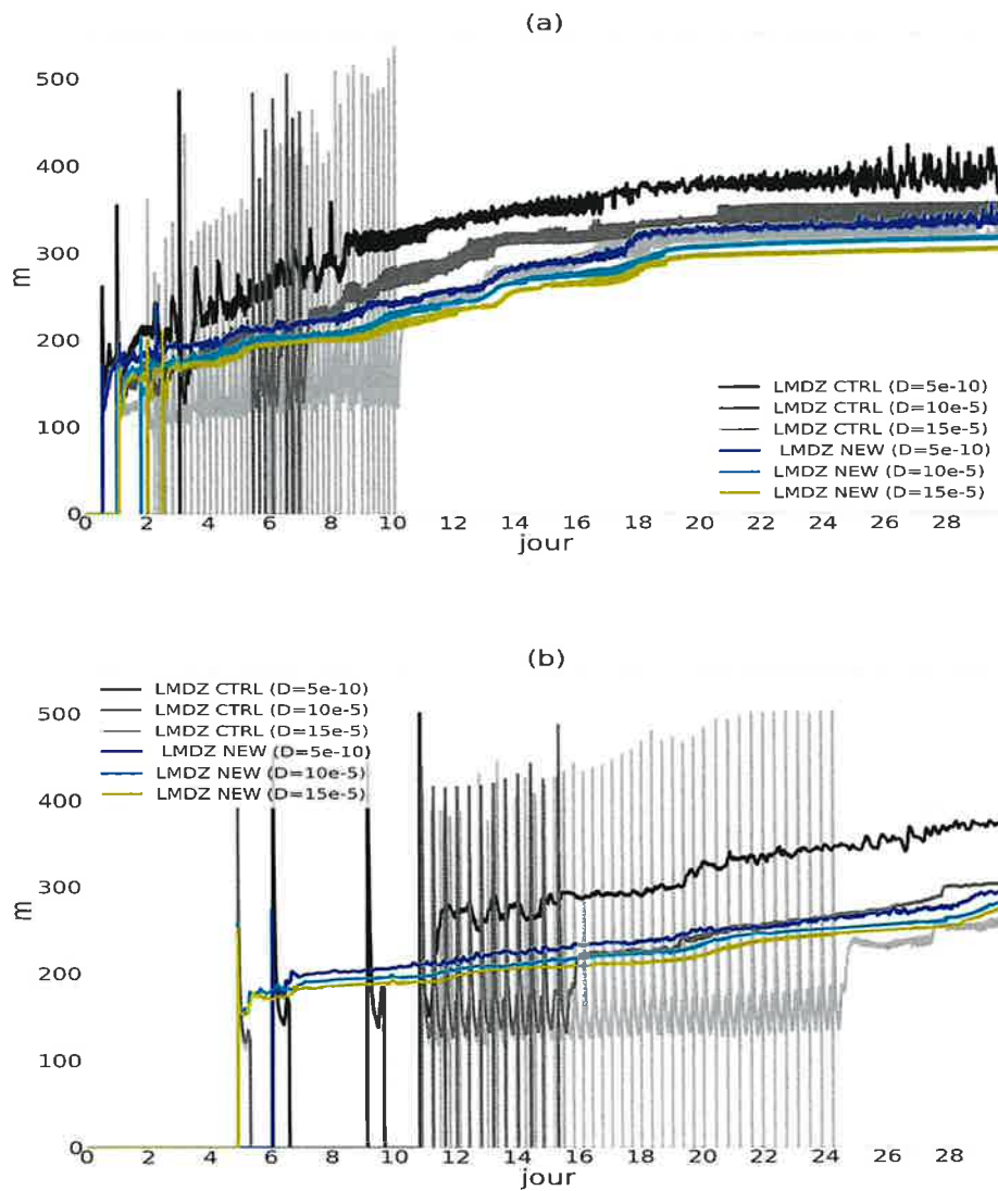
FIGURE 1.10 Comparaison de la hauteur des poches ( h_{wk} ) dans LMDZ selon l'ancien et le nouveau schéma numérique pour le calcul de h_{wk} (correspondant respectivement à LMDZ CTRL et LMDZ NEW), avec une densité fixée à D_{wk} = 5^{-10} , D_{wk} = 10^{-10} et D_{wk} = 15^{-10} , pour des pas de temps de 10 minutes (a) et de 5 minutes (b).
