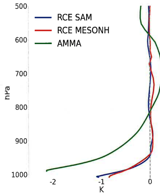
FIGURE 1.6 Profils verticaux de l'écart de température entre l'intérieur et l'extérieur des poches froides calculés sur un instant des LES (SAM et MESONH) du cas RCE et un instant de la LES MESONH du cas AMMA.
