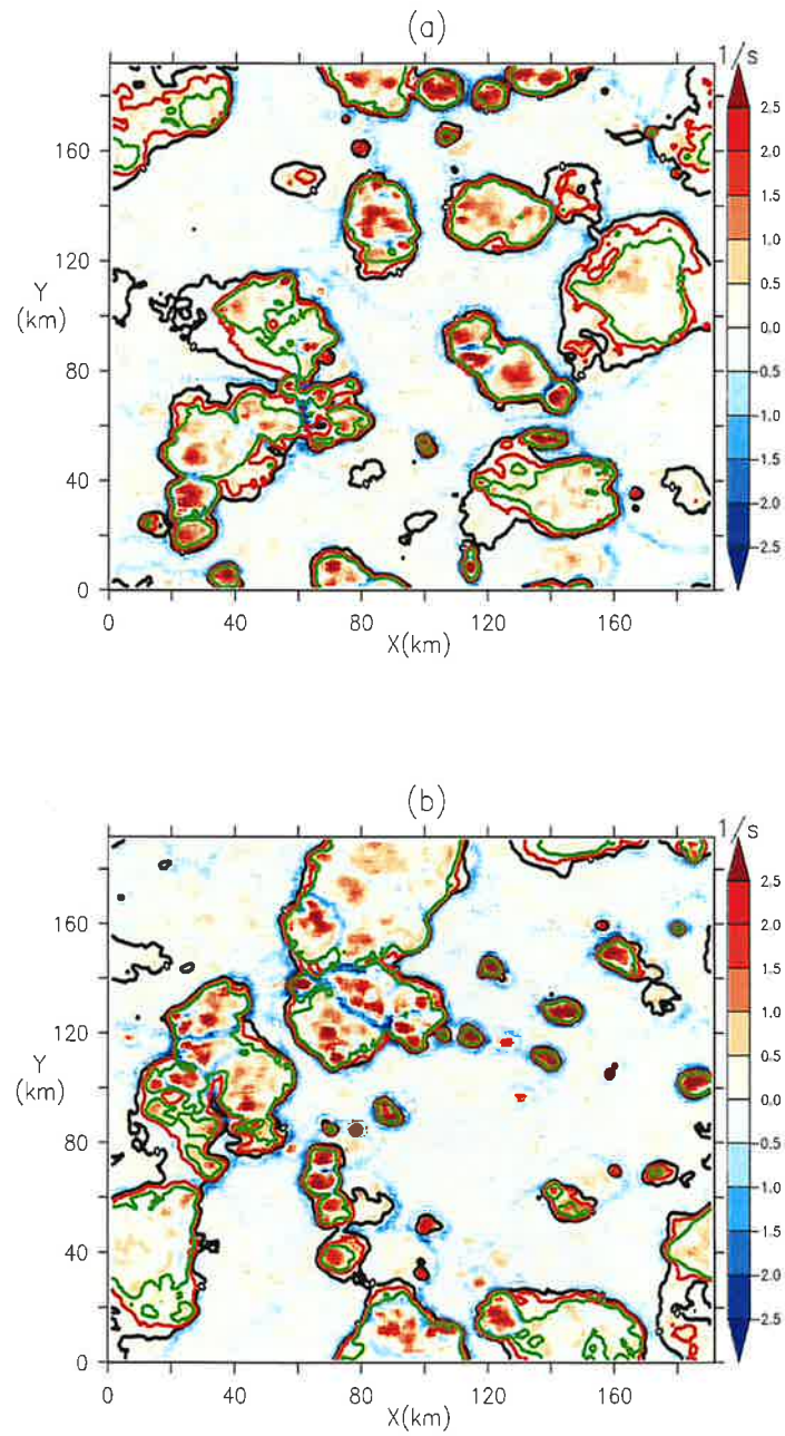
FIGURE 1.2 Carte de la divergence du vent à 10 m (en s^{-1} ) multipliée par 1000 et lissée horizontalement sur 3.25 \text{ km} \times 3.25 \text{ km} représentée sur deux instants (a et b) de la LES SAM réalisée sur le cas RCE océanique et superposés avec les contours d'anomalies de températures à 10 m à -0.4 \text{ K} (vert), -0.2 \text{ K} (rouge) et 0 \text{ K} (noir)
