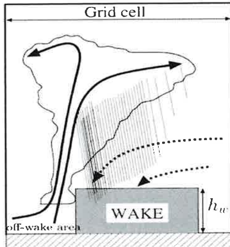
FIGURE 1.1 Schéma conceptuel d'un courant de densité (Grandpeix and Lafore, 2010).
