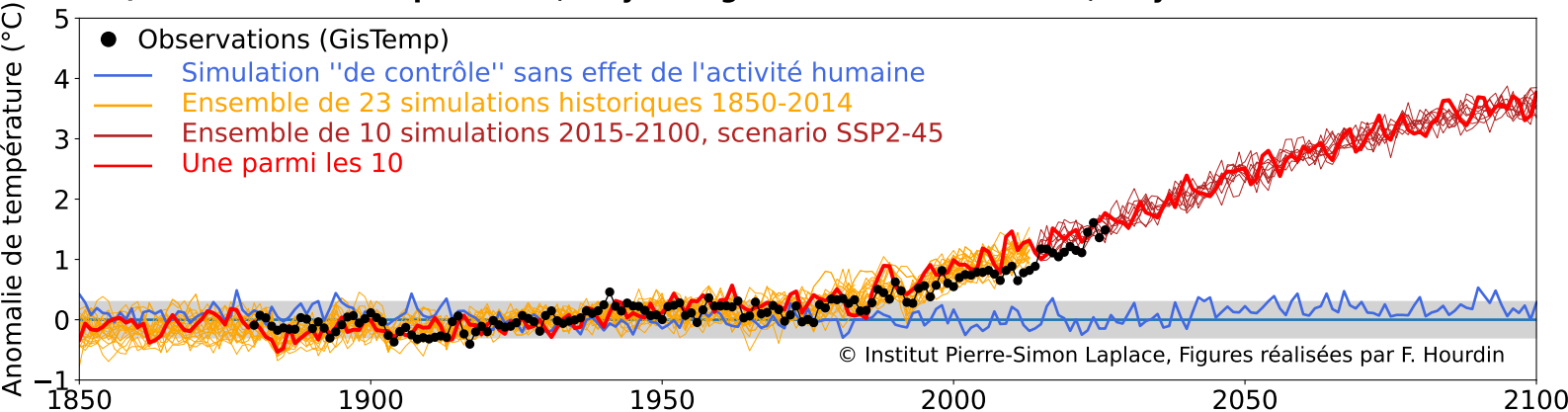
b) Evolution des températures, France métropolitaine, juin-juillet-août
