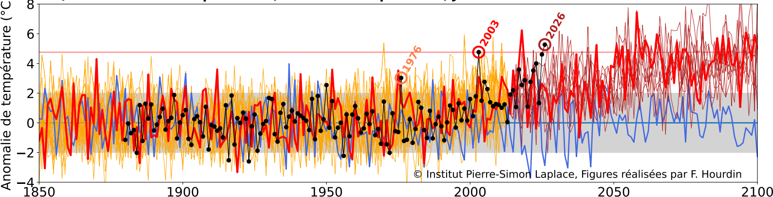
c) Evolution des températures, France métropolitaine, juin
