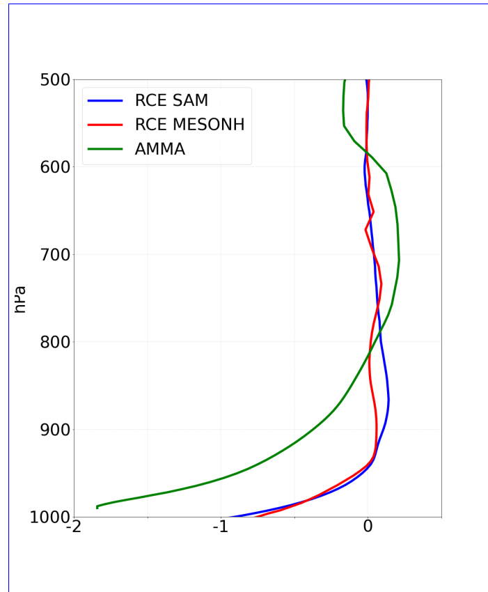
Figure 4: Vertical profiles of the temperature difference between the inside and the outside of cold pools calculated at an instant of the LES (SAM and MESONH) of the RCE case and an instant of the LES MESONH of the AMMA case. Ajouter l'heure et peut être mettre les deux heures ? Peut être mettre aussi plusieurs courbes pour les RCE. Une dizaine chacune ?
