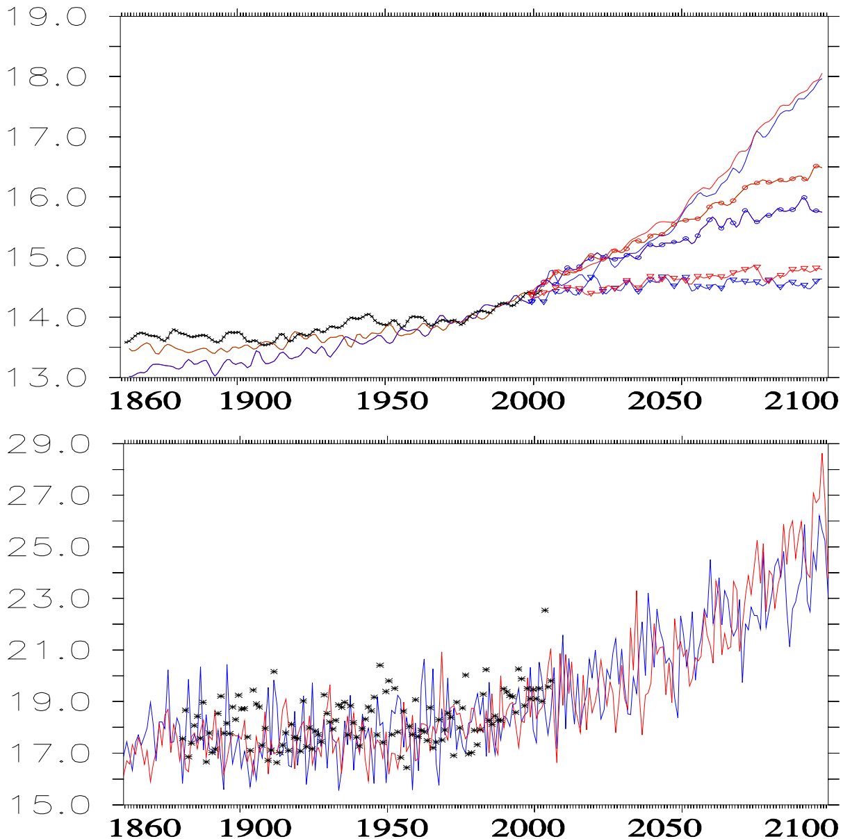
Figure 1: En haut : Evolution de la température moyenne de surface du globe (°C) observée (en noir, de 1860 à 2004), et simulée par les modèle du CNRM (en bleu) et de l'IPSL (en rouge). Après l'an 2000, on utilise soit le scénario SRES-A2 (trait continu), soit le scénario SRES-B1 (trait avec cercle), soit on maintient la concentration de CO2 constante (trait avec triangle). Les observations sont celles compilées par le CRU [Jones et Moberg, 2003]. En bas : Evolution de la température moyenne (°C) durant les 3 mois d'été (juin à août) en France métropolitaine observée (en noir, de 1880 à 2005), et simulée par les modèle du CNRM (en bleu) et de l'IPSL (en rouge). Après l'an 2000, on utilise le scénario SRES-A2. L'été 2003 est bien visible. Les observations proviennent de Météo France (Moisselin et al, 2002).
