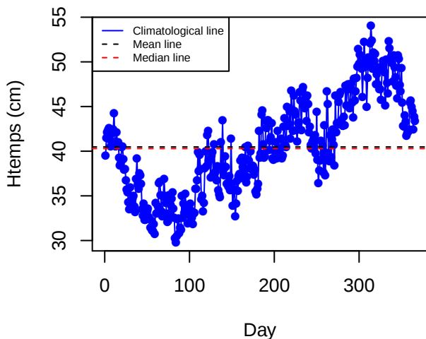
Climatology (GMLD)
