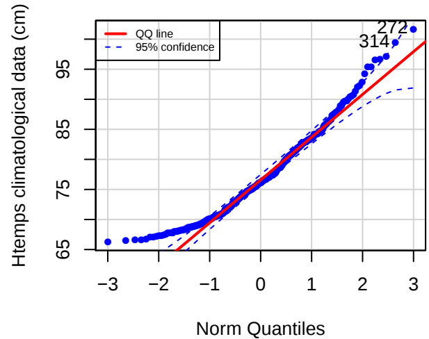
QQ plot (GMPL)
