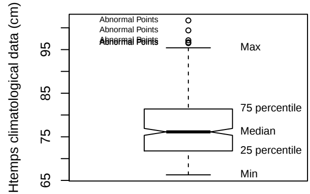
Box plot (GMPL)
