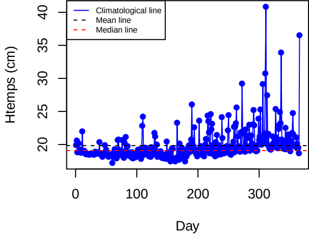
Climatology (LAMC)
