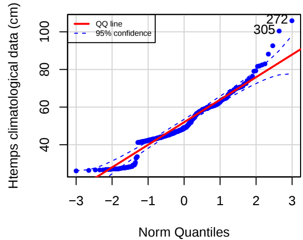
QQ plot (LAML)
