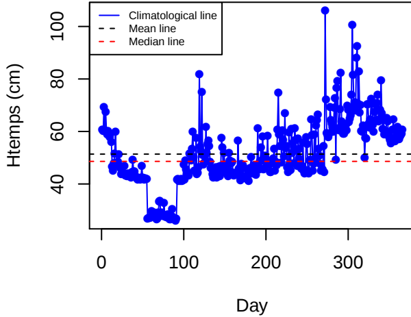
Climatology (LAML)
