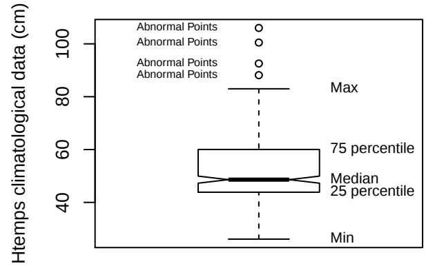
Box plot (LAML)
