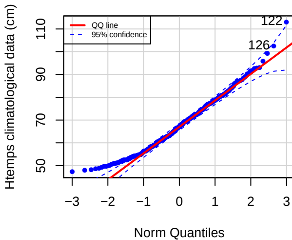
QQ plot (LAMP)
