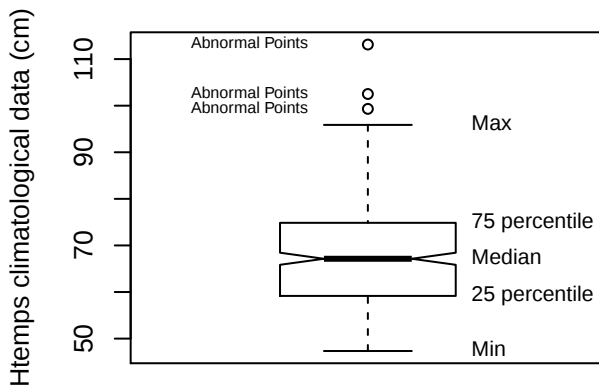
Box plot (LAMP)
