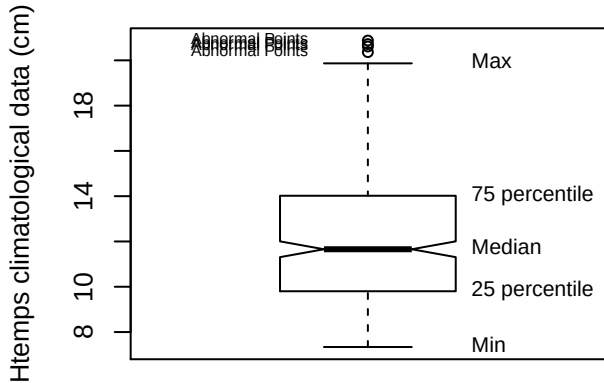
Box plot (STJA)
