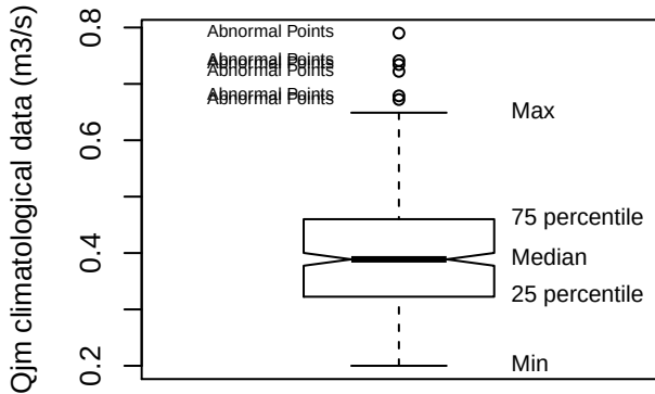
Box plot (GMLP)
