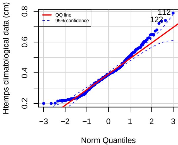
QQ plot (GMLP)
