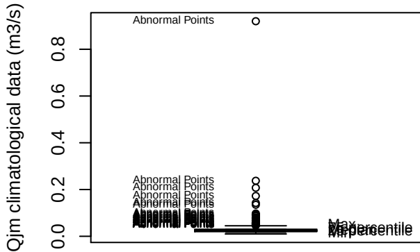
Box plot (LAMC)
