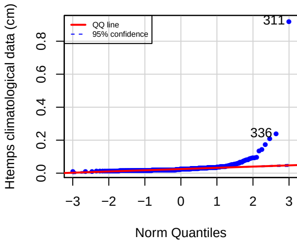
QQ plot (LAMC)
