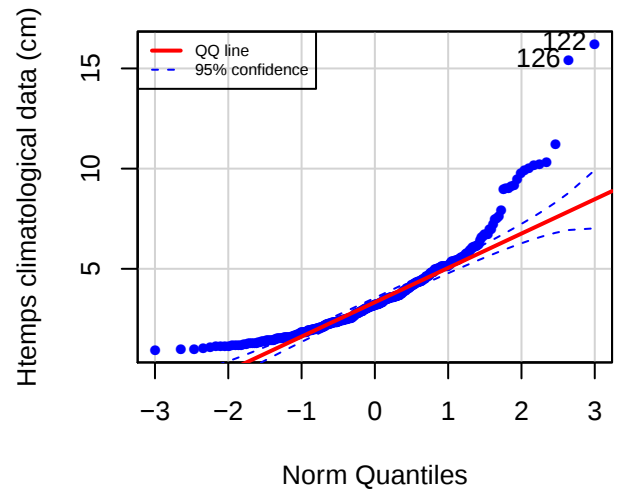
QQ plot (LAMP)
