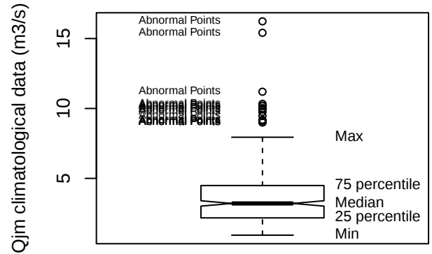
Box plot (LAMP)
