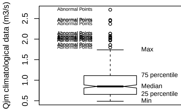
Box plot (STJA)
