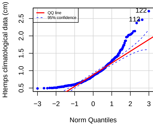
QQ plot (STJA)
