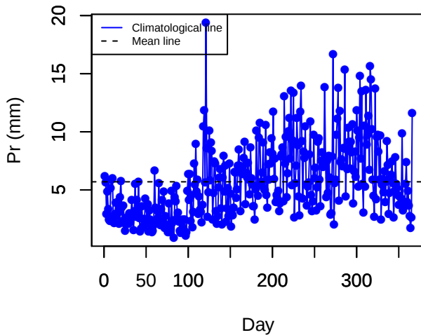
Climatology (LAMA)
