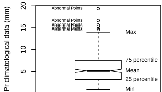
Box plot (LAMA)
