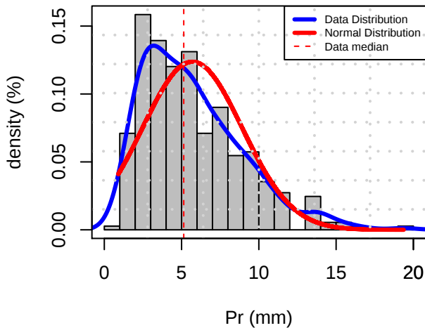
Histogram Distribution (LAMA)
