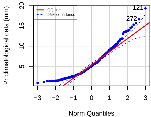
QQ plot (LAMA)
