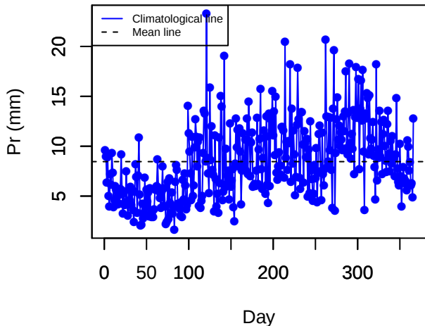
Climatology (STJO)
