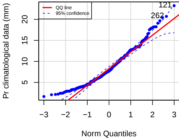
QQ plot (STJO)
