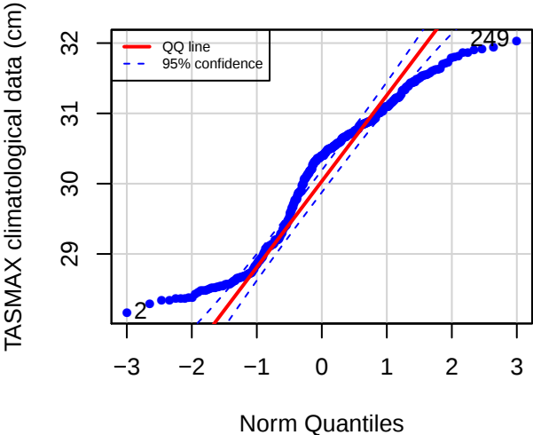
QQ plot (DUCO)
