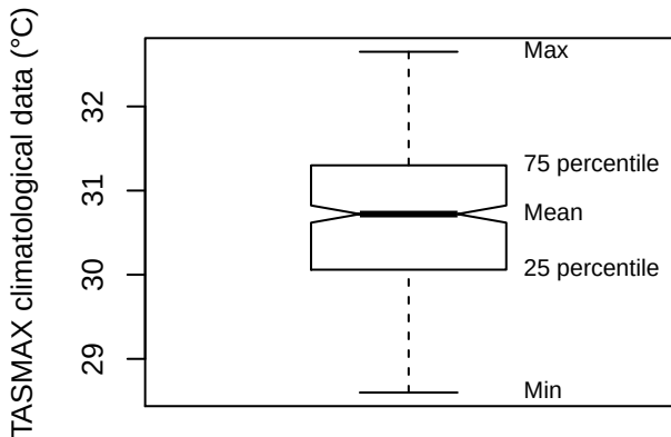
Box plot (PANS)
