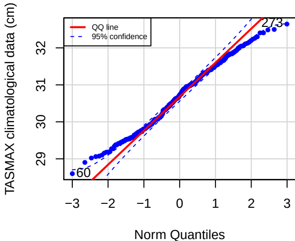
QQ plot (PANS)
