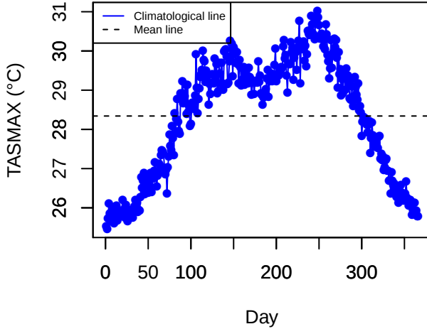
Climatology (STJO)
