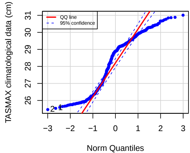
QQ plot (STJO)
