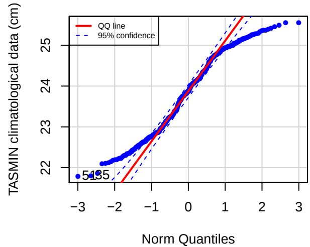
QQ plot (DUCO)
