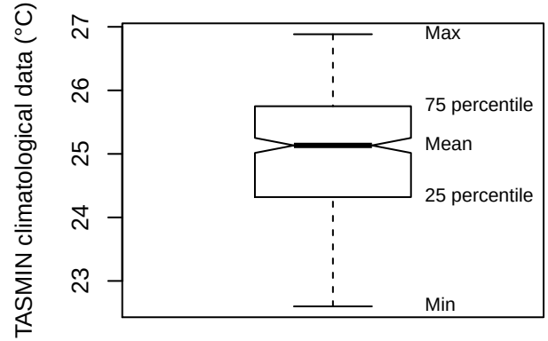
Box plot (PANS)
