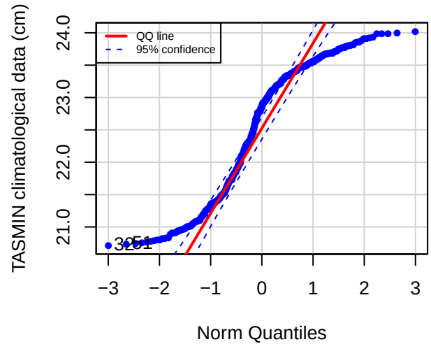
QQ plot (STJO)
