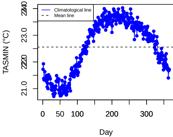
Climatology (STJO)
